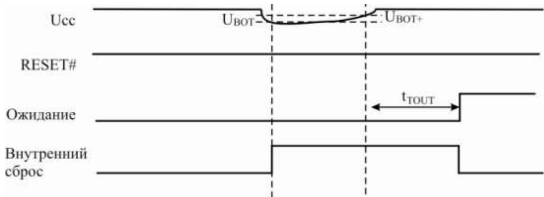
Рисунок 3.17 – Сброс по отключению питания во время работы
