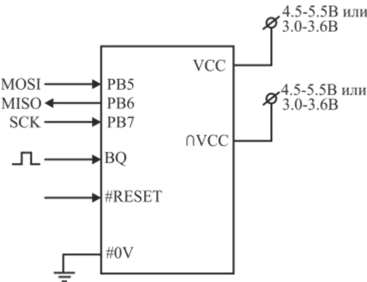
Рисунок 3.118 – Включение схемы при последовательном программировании и верификации
