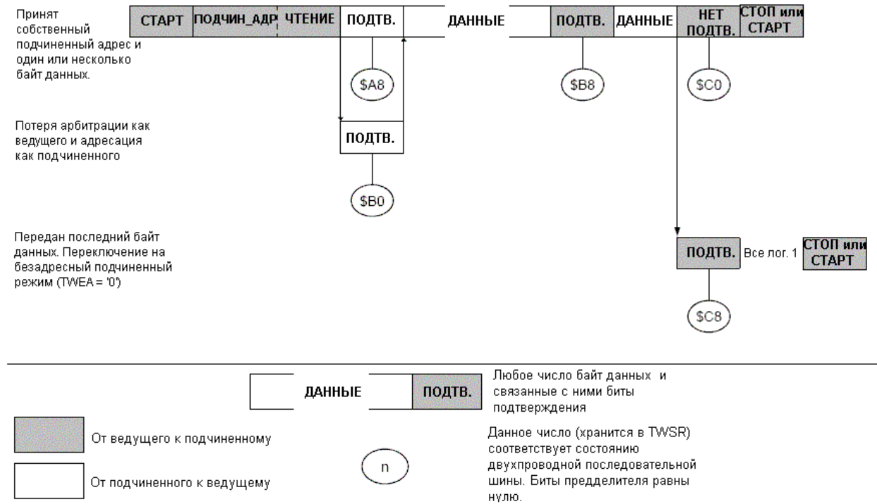
Рисунок 3.91 – Форматы и состояния в режиме подчиненного передатчика
