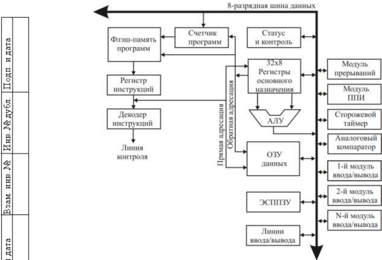
Рисунок 3.1 – Блок-схема архитектуры ядра микропрограммного управления
