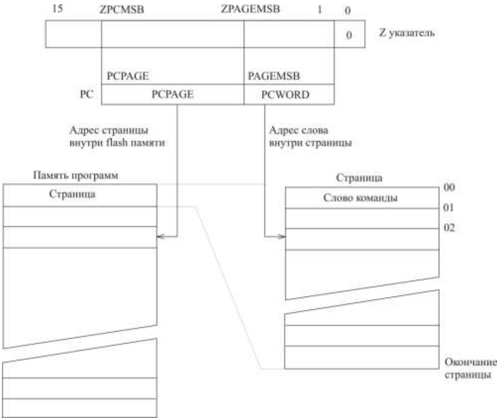
Рисунок 3.109 – Адресация к памяти программ через Z-указатель
