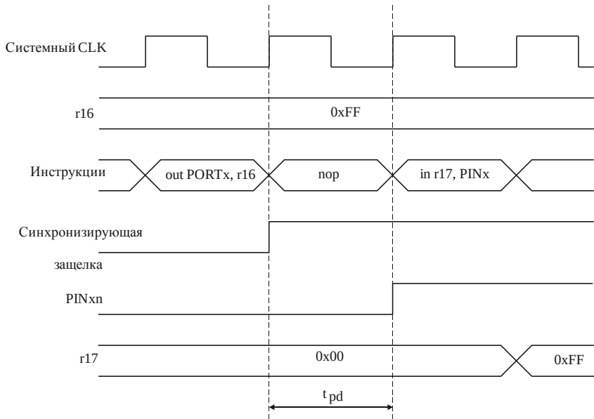
Рисунок 3.23 – Синхронизация при считывании значения вывода, определенного программно
