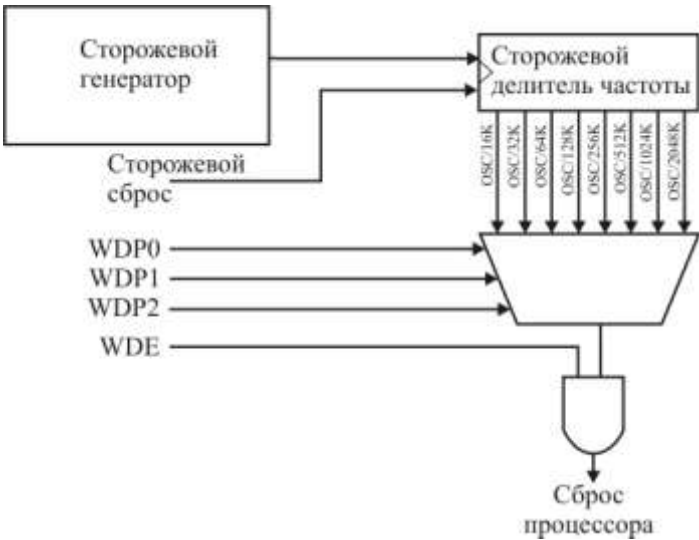
Рисунок 3.19 – Сторожевой таймер
