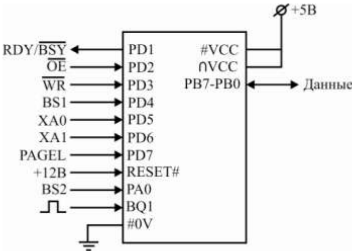
Рисунок 3.110 – Включение схемы при параллельном программировании
