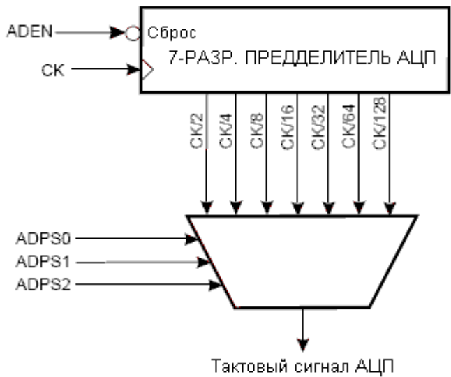
Рисунок 3.98 Предделитель АЦП
