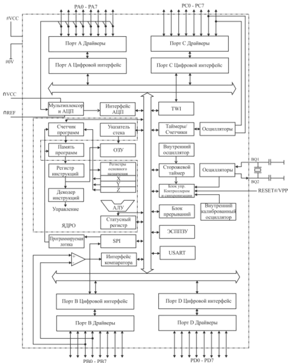
Рисунок 2.1 – Структурная схема ИС 1887ВЕ4У
