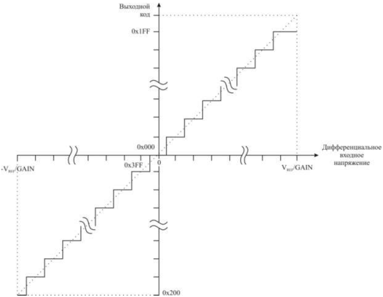
Рисунок 3.108 – Функция преобразования АЦП при измерении дифференциального сигнала
