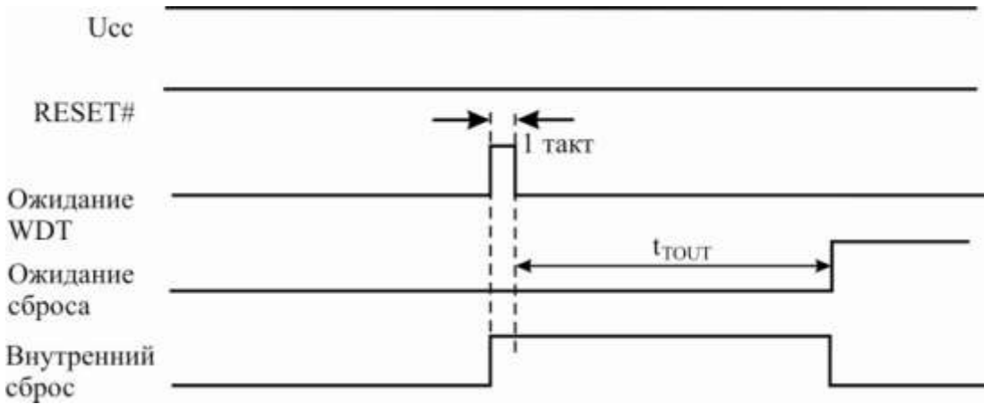
Рисунок 3.18 – Сброс от сторожевого таймера во время работы
