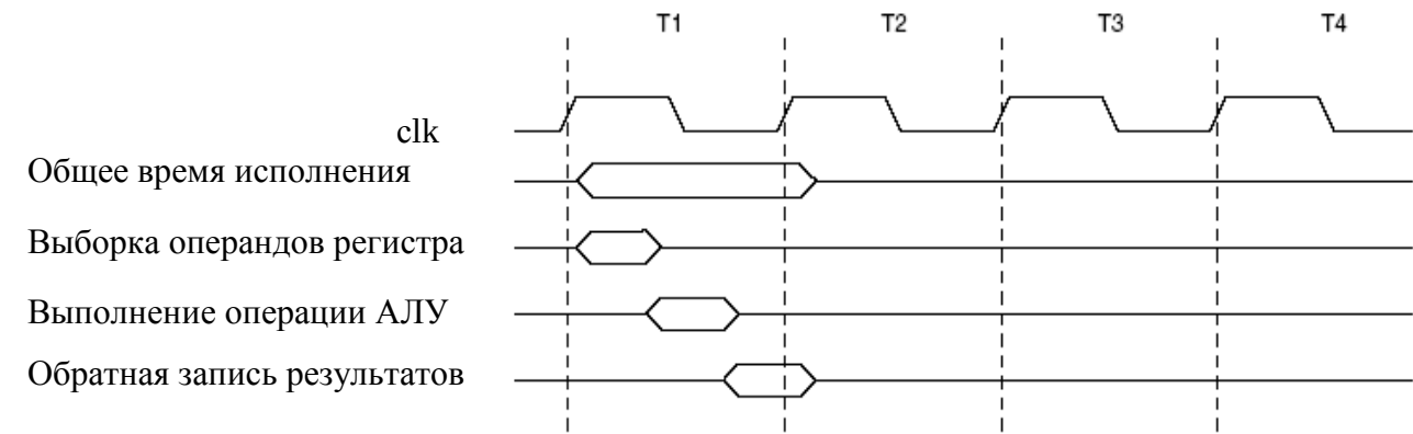
Рисунок 3.5 – Работа АЛУ в одиночном цикле
