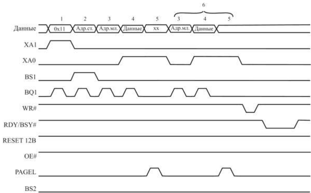
Рисунок 3.112 – Временная диаграмма программирования массива EEPROM
