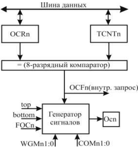
Рисунок 3.53 – Блок-схема модуля сравнения выхода
