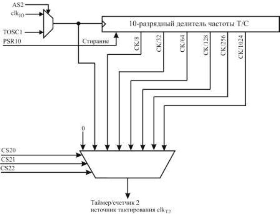
Рисунок 3.62 – Предделитель таймера/счетчика 2
