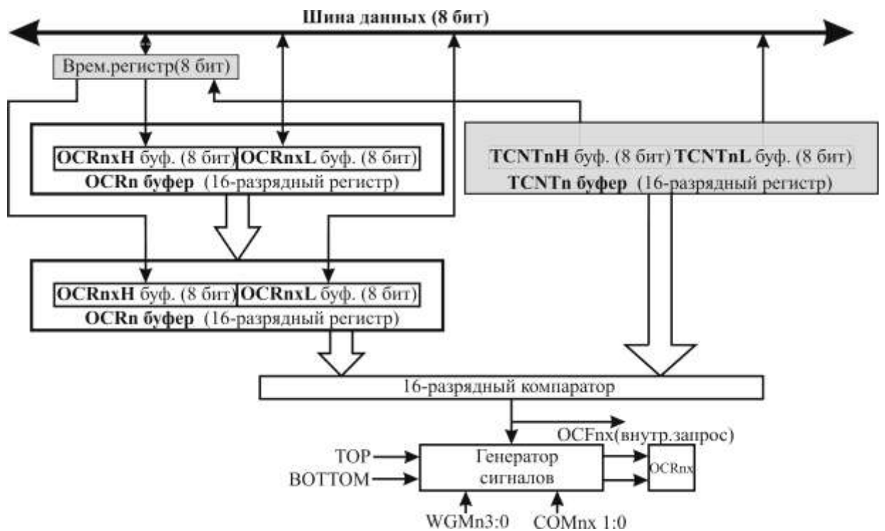
Рисунок 3.41 – Блок-схема модуля сравнения по выходу
