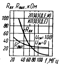
Зависимости входного и выходного сопротивлений от частоты
