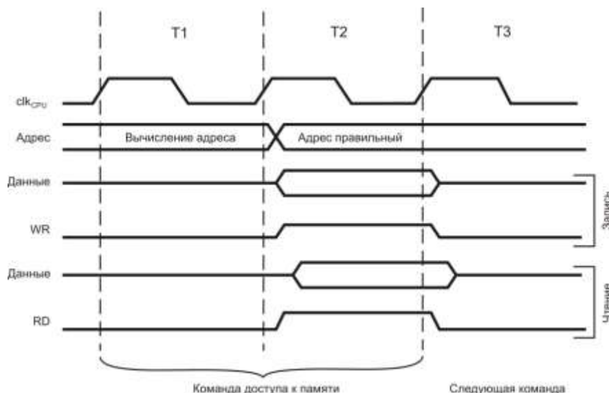
Рисунок 3.11 – Циклы доступа к данным статического ОЗУ на кристалле
