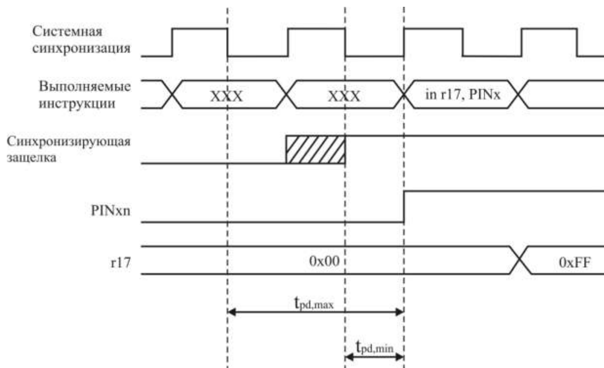
Рисунок 3.32 – Синхронизация при считывании внешне приложенного к выводу уровня
