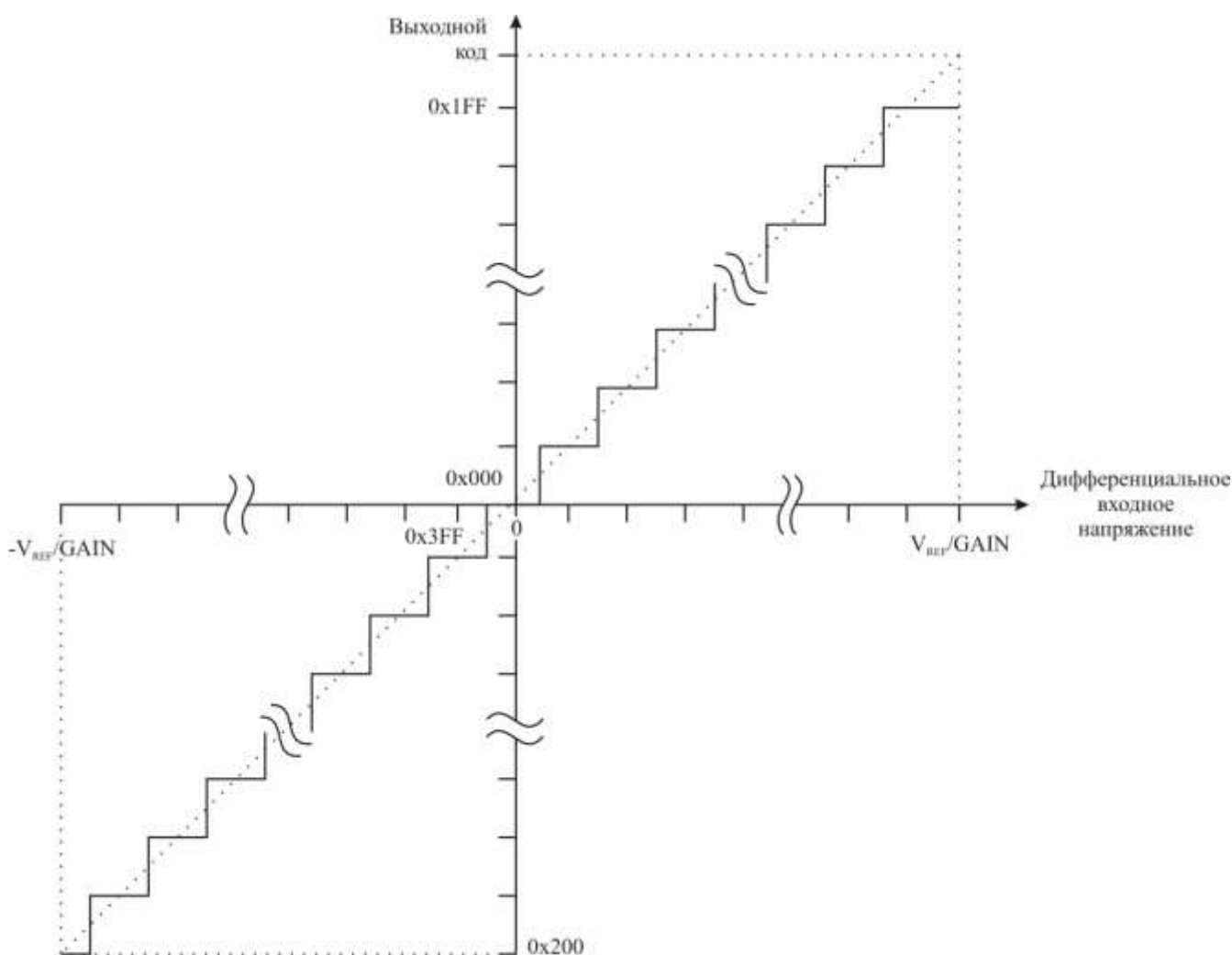
Рисунок 3.120 – Функция преобразования АЦП при измерении дифференциального сигнала
