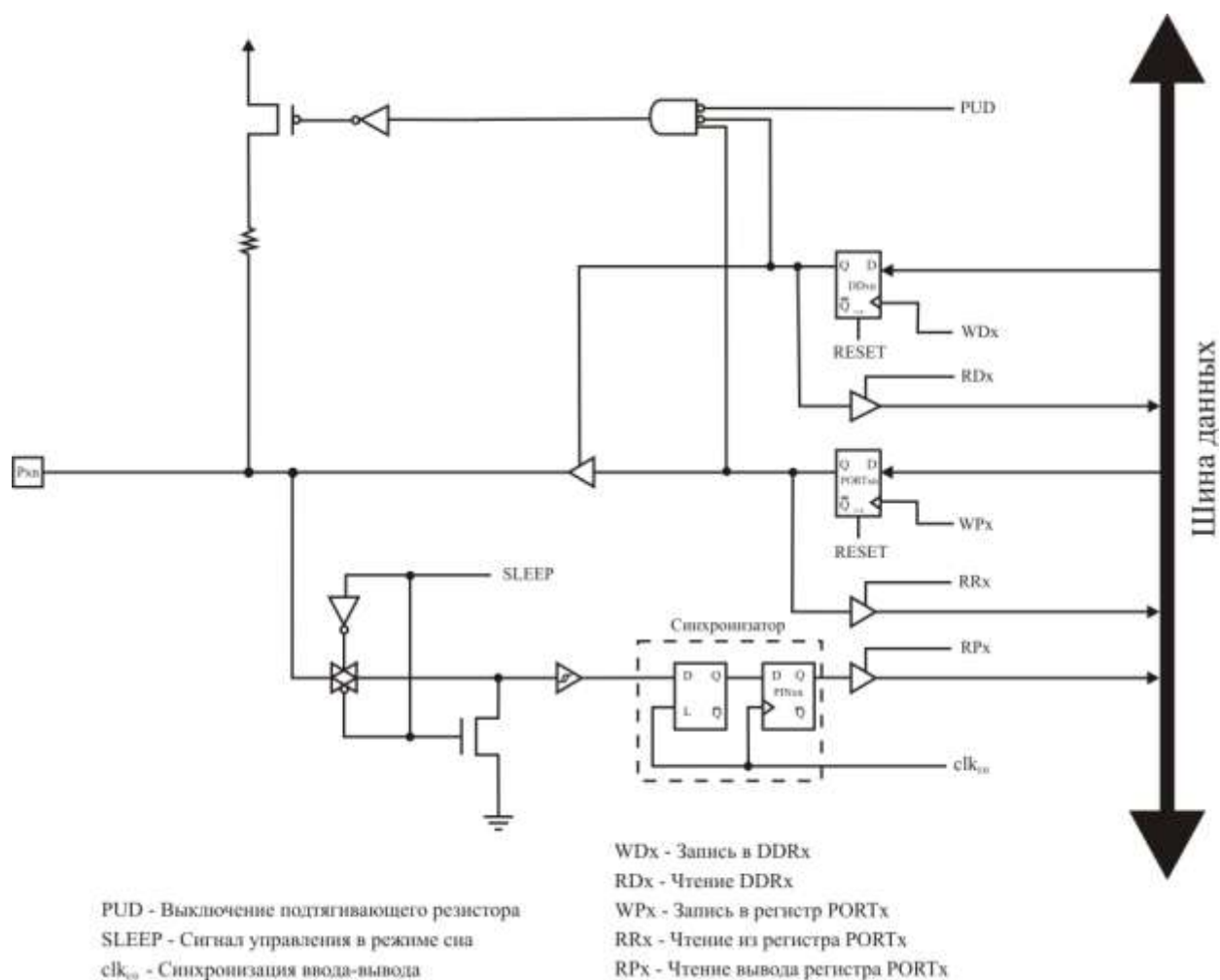
Рисунок 3.31 – Организация общего цифрового ввода-вывода
