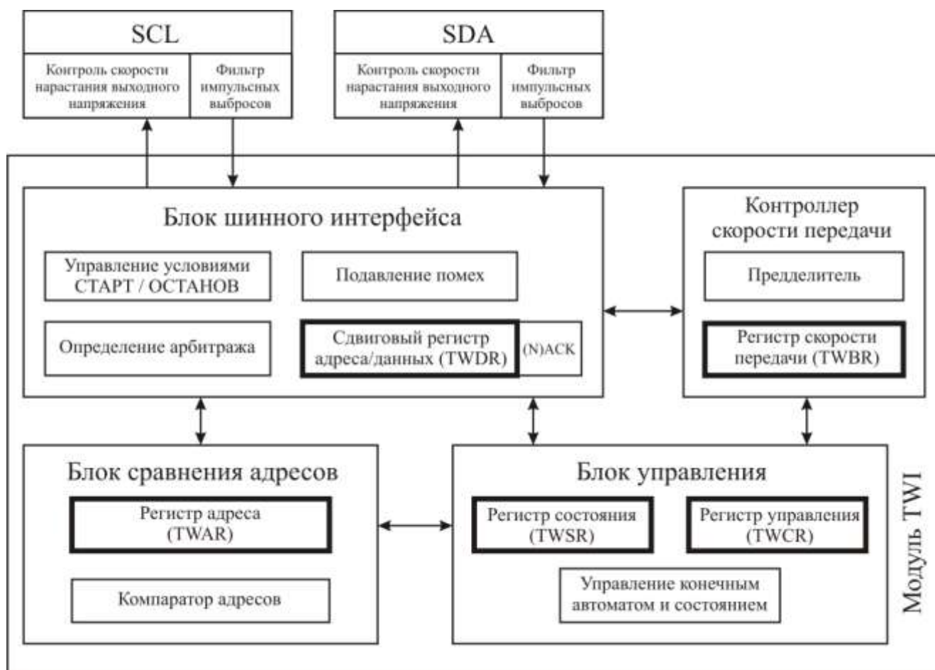
Рисунок 3.95 – Структурная схема модуля TWI
