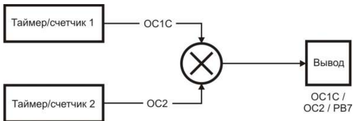
Рисунок 3.73 – Блок-схема модулятора сравнения
