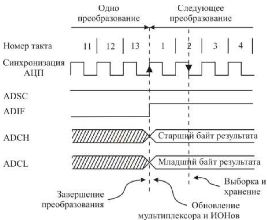
Рисунок 3.113 – Временная диаграмма работы АЦП в автономном режиме
