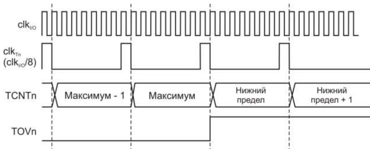
Рисунок 3.43 – Временная диаграмма таймера/счетчика с делением ( f_{clk\_I/O}/8 )
