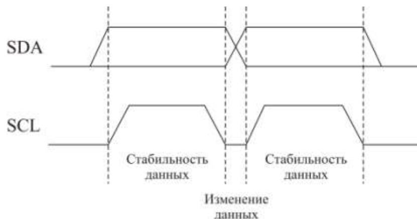
Рисунок 3.88 – Действительность данных
