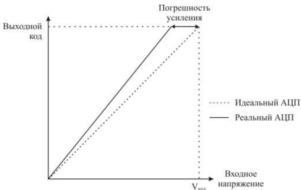
Рисунок 3.117 – Погрешность усиления
