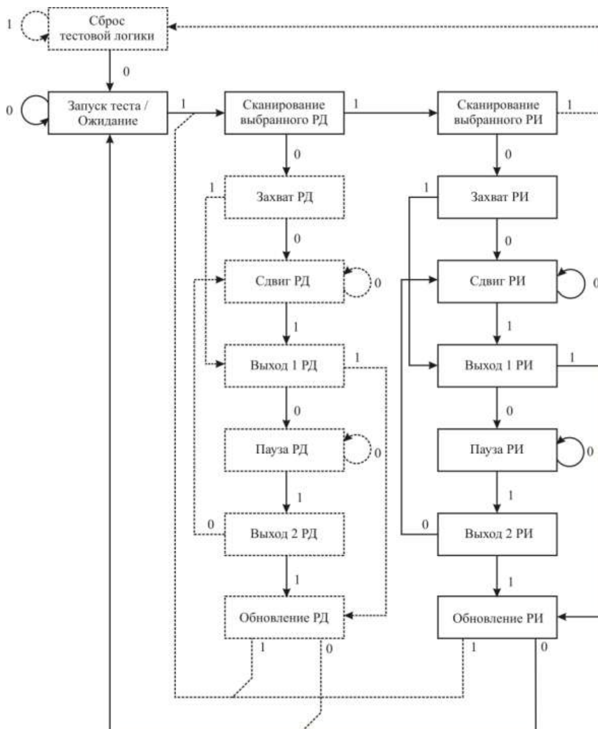
Рисунок 3.147 – Последовательность конечного автомата для изменения слова инструкции
