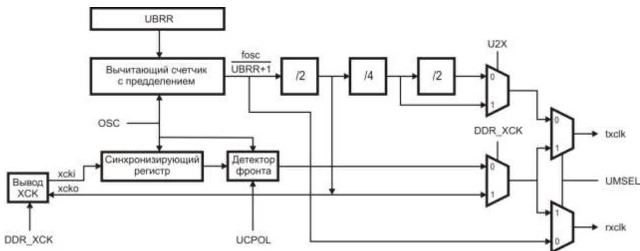
Рисунок 3.81 – Структурная схема логики генерации тактовых импульсов
