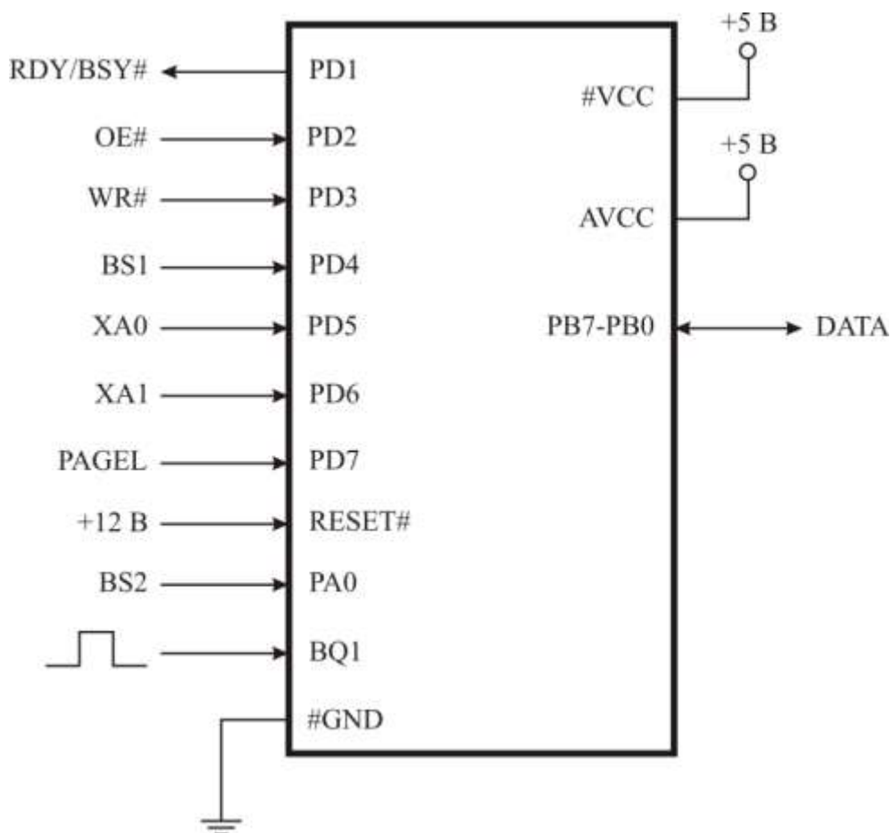
Рисунок 3.136 – Параллельное программирование
