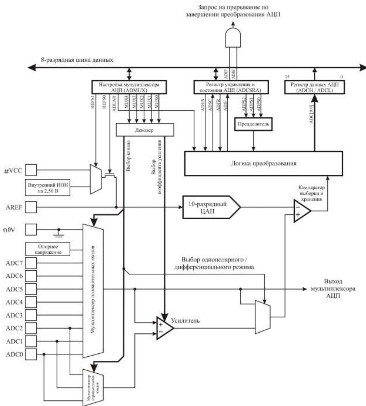
Рисунок 3.109 – Структурная схема АЦП
