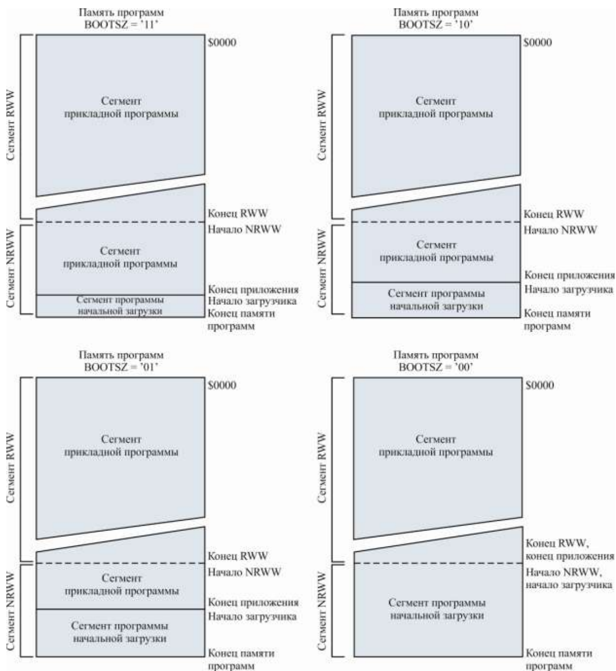
Рисунок 3.134 – Сегменты памяти
