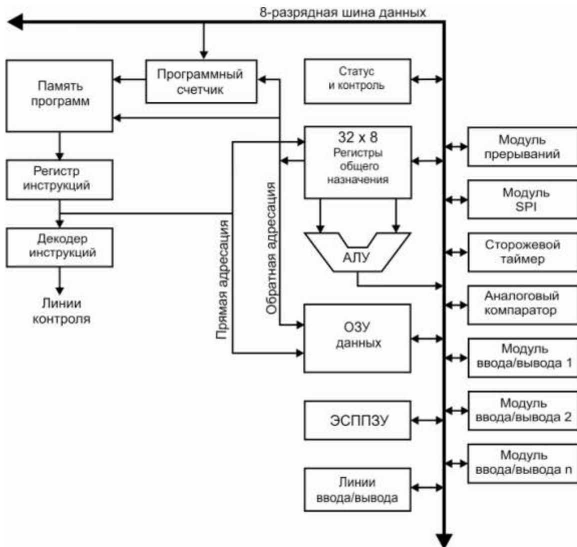
Рисунок 3.1 – Блок-схема архитектуры ядра микропрограммного управления
