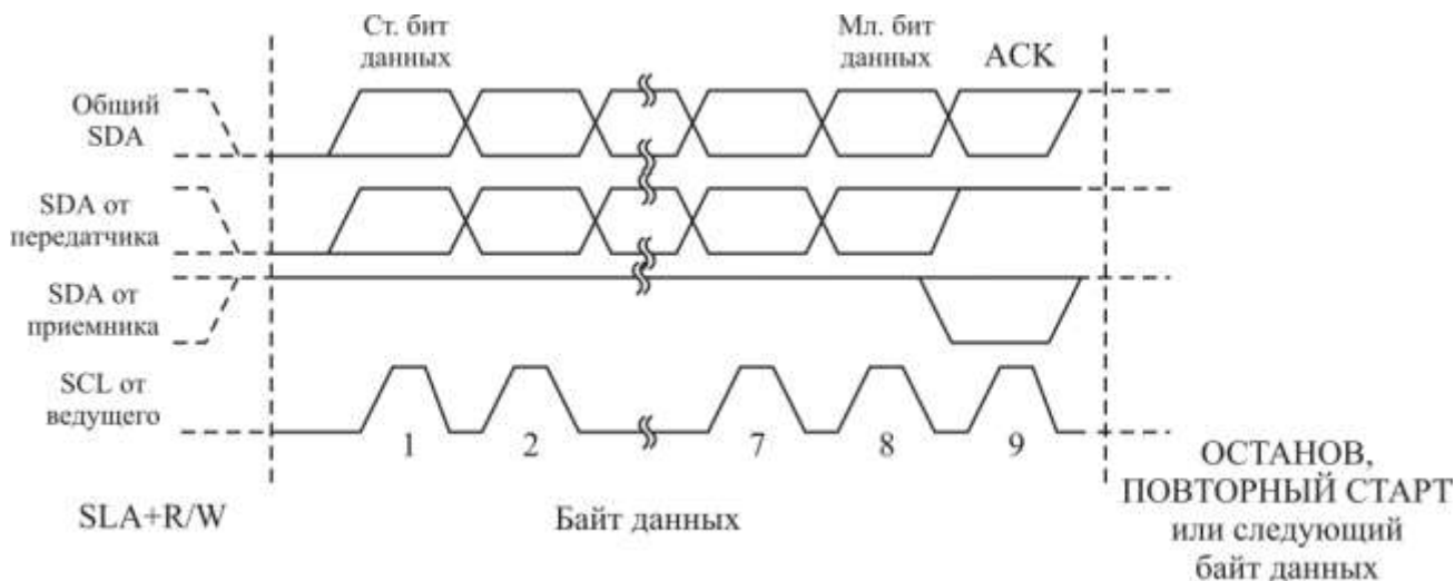
Рисунок 3.91 – Формат пакета данных
