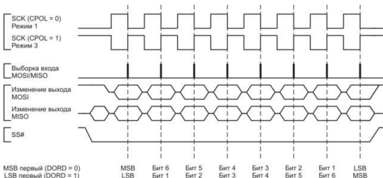
Рисунок 3.79 – Временная диаграмма передачи данных, когда CPHA = 1
