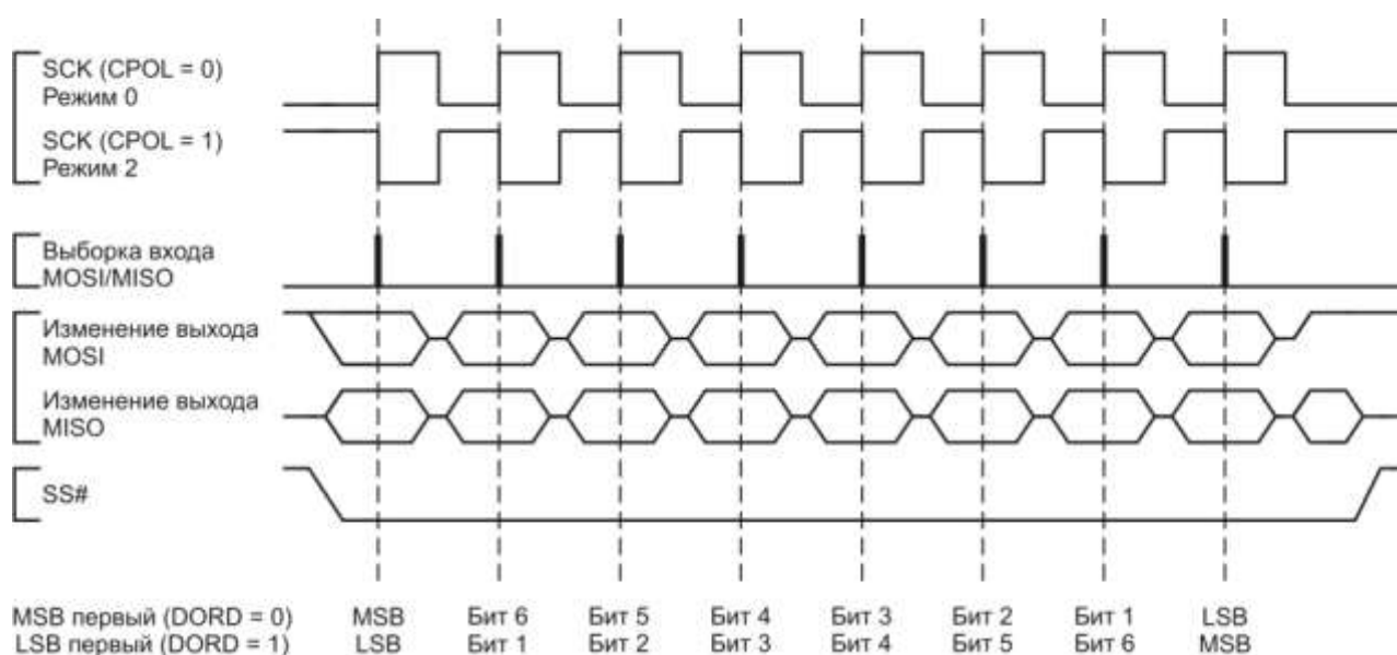
Рисунок 3.78 – Временная диаграмма передачи данных, когда CPHA = 0
