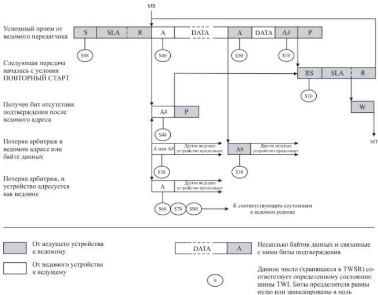
Рисунок 3.100 – Форматы и состояния в режиме ведущего приемника
