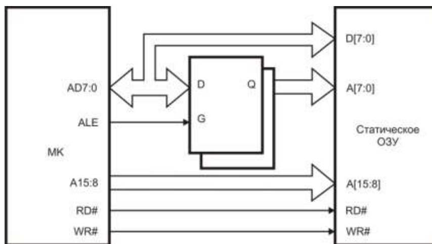
Рисунок 3.13 – Подключение внешнего статического ОЗУ к AVR-микроконтроллеру
