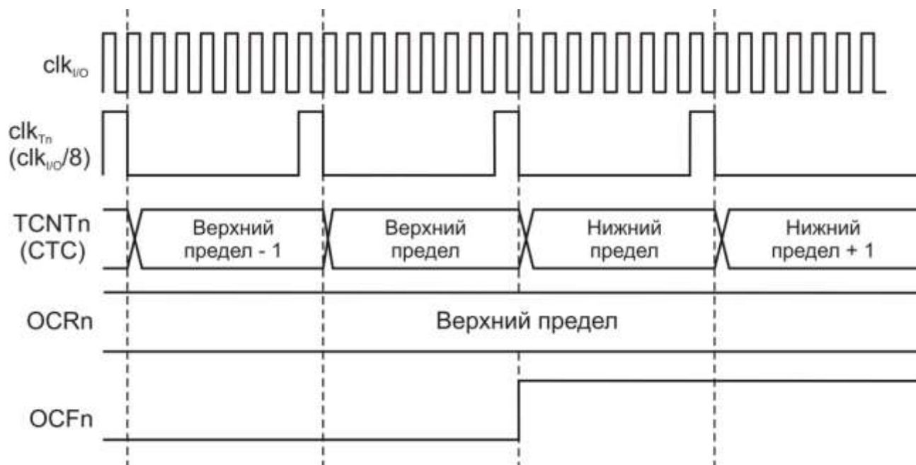
Рисунок 3.72 – Временная диаграмма таймера/счетчика, с предделением ( f_{clk\_I/O}/8 ), в режиме сброса таймера при совпадении
