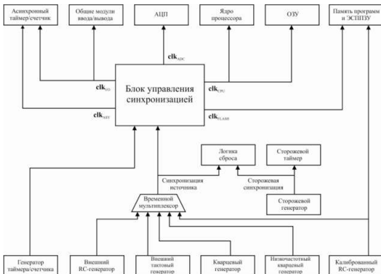
Рисунок 3.19 – Распределение тактовых импульсов
