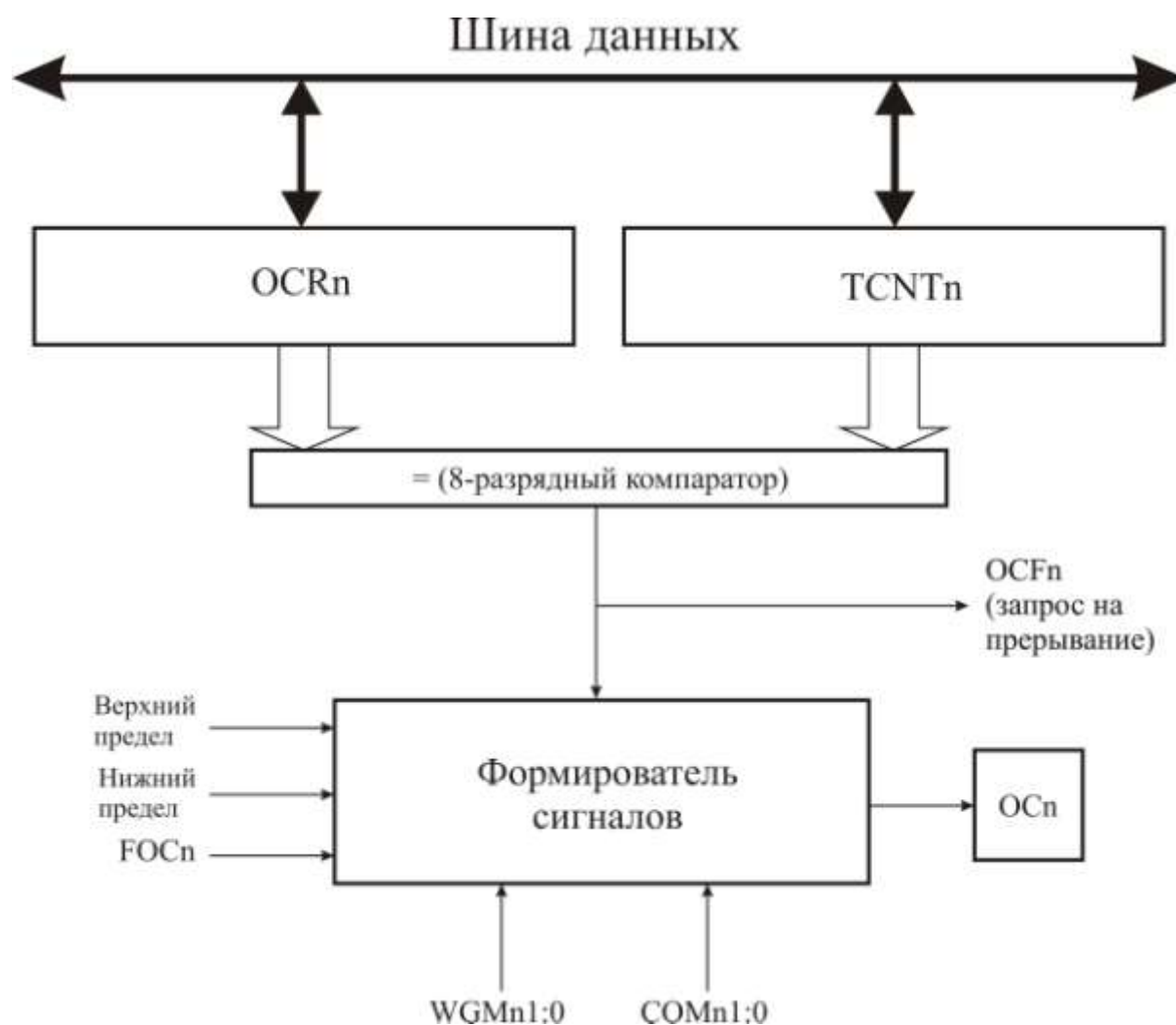
Рисунок 3.37 – Структурная схема блока сравнения
