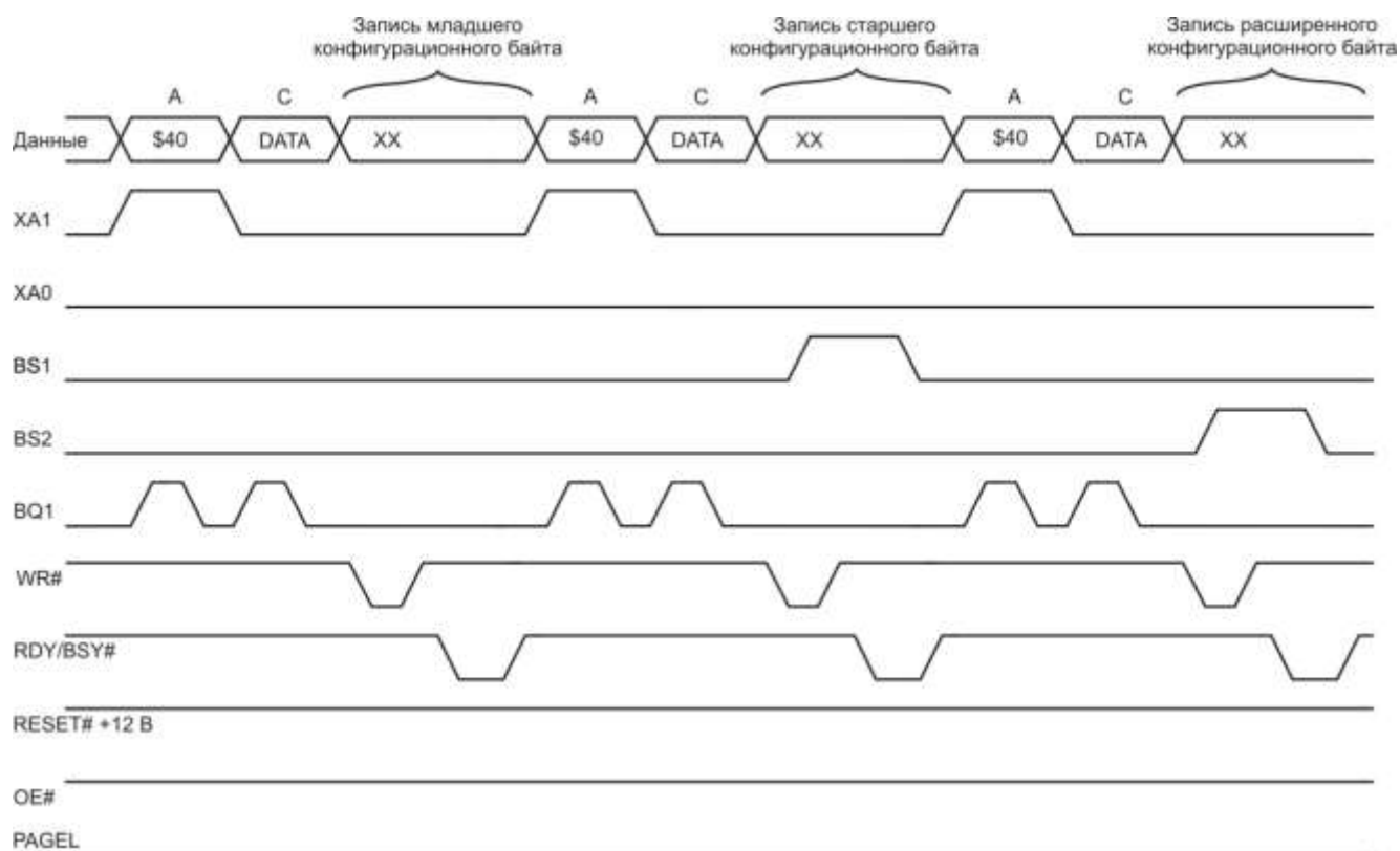
Рисунок 3.140 – Программирование конфигурационных битов
