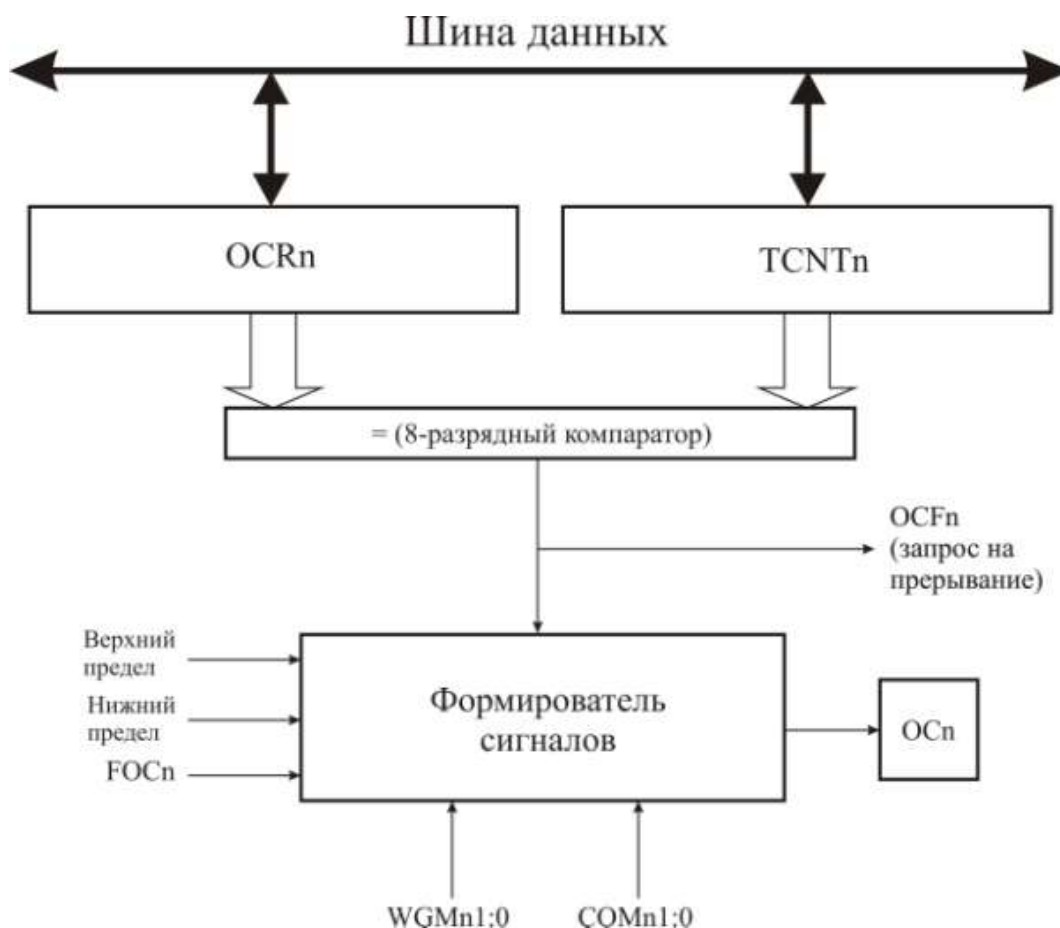
Рисунок 3.64 – Структурная схема блока сравнения
