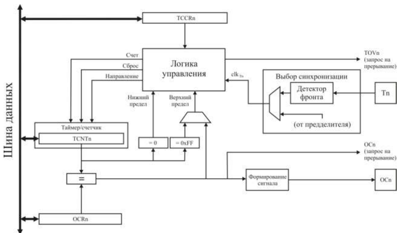
Рисунок 3.62 – Структурная схема 8-разрядного таймера/счетчика 2
