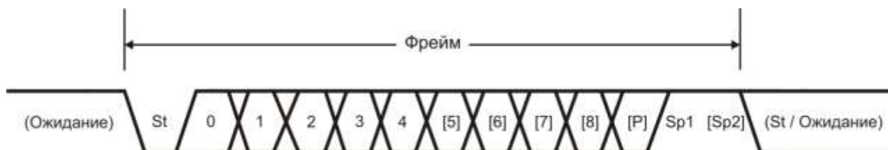
Рисунок 3.83 – Форматы фреймов
