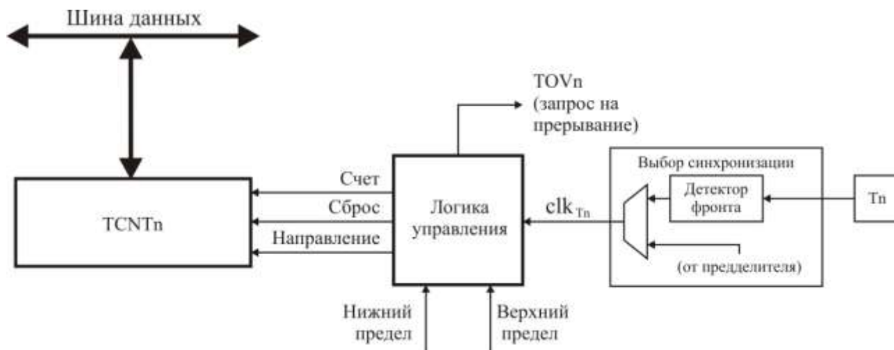
Рисунок 3.63 – Структурная схема блока счетчика
