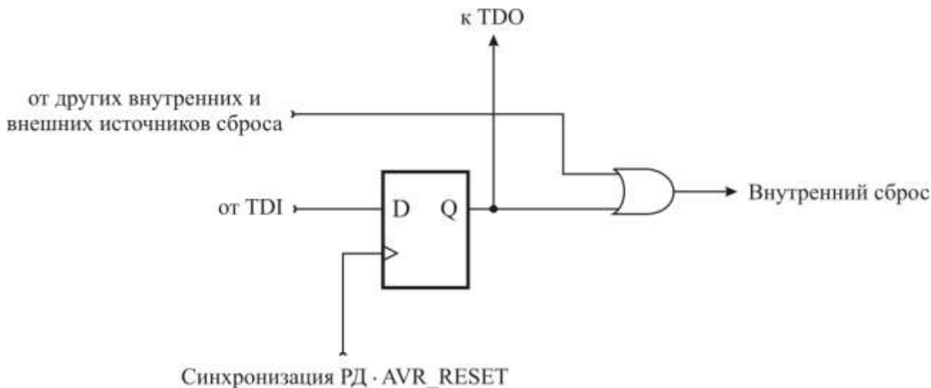
Рисунок 3.124 – Регистр сброса
