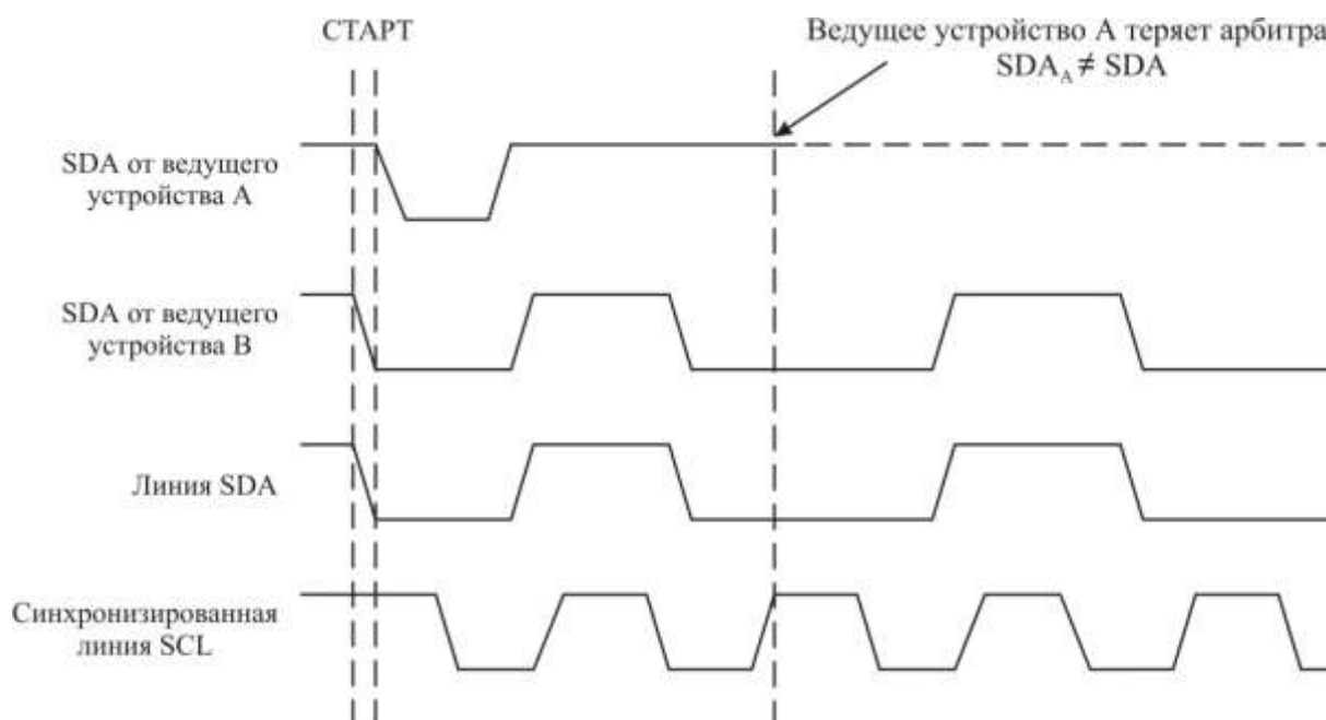
Рисунок 3.94 – Арбитраж между двумя ведущими устройствами
