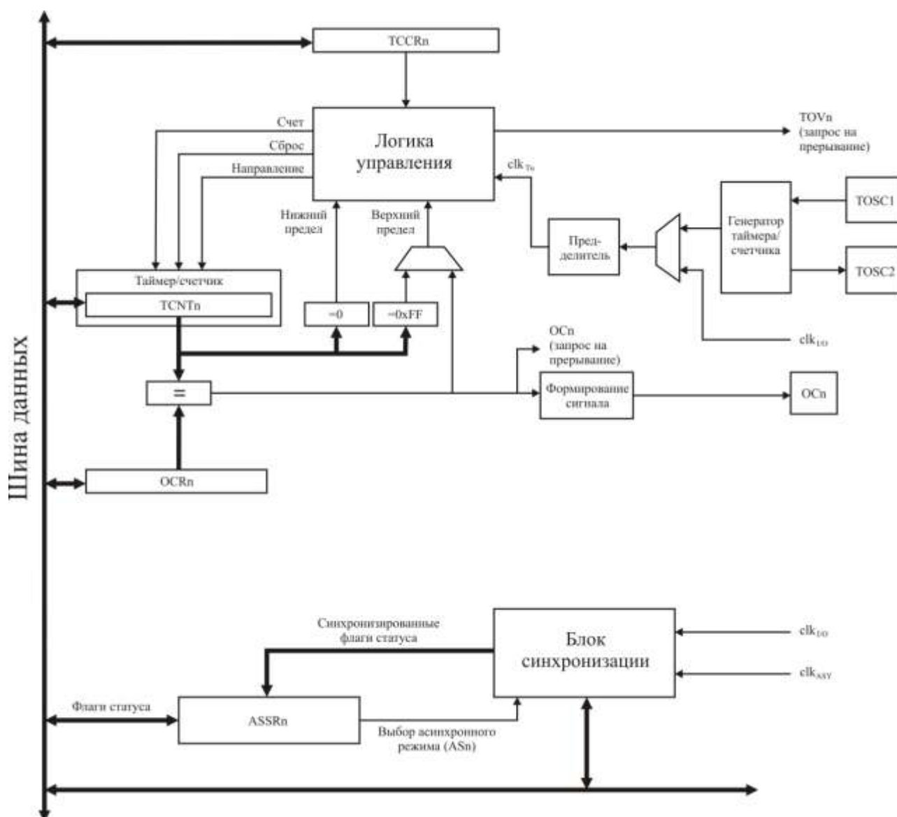
Рисунок 3.35 – Структурная схема 8-разрядного таймера/счетчика 0
