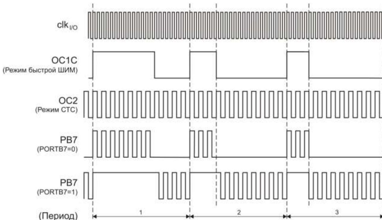
Рисунок 3.75 – Временная диаграмма работы модулятора сравнения
