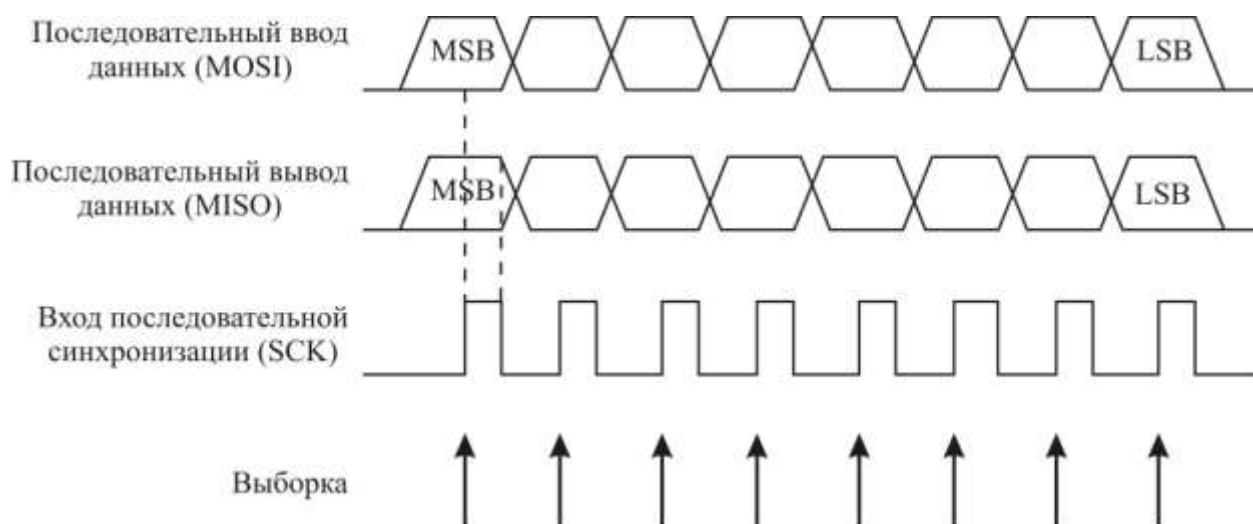
Рисунок 3.146 – Формы сигналов при последовательном программировании через SPI
