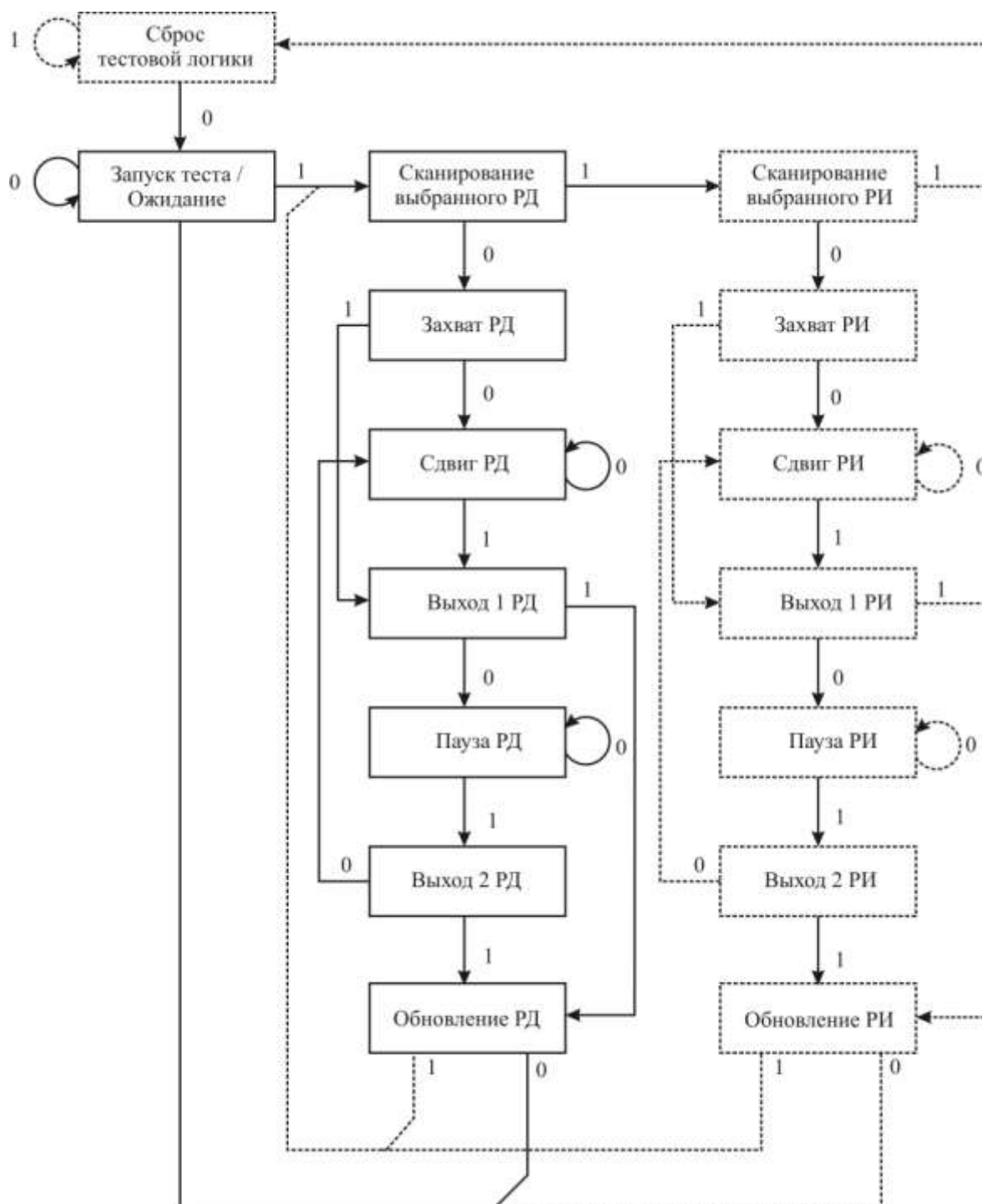
Рисунок 3.150 – Последовательность конечного автомата для изменения/чтения слова данных
