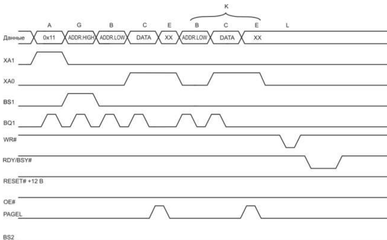
Рисунок 3.139 – Программирование форм сигналов для ЭСППЗУ
