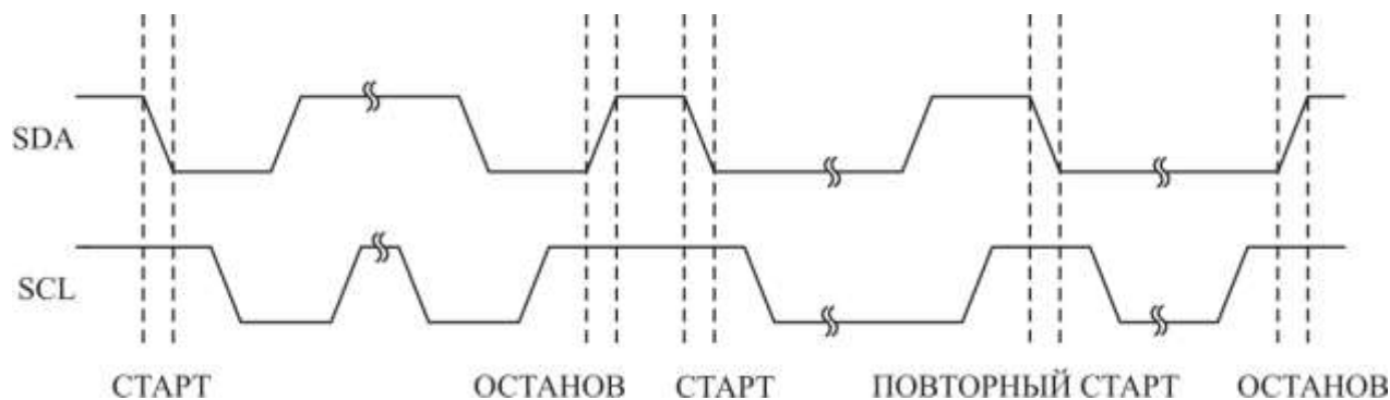
Рисунок 3.89 – Условия СТАРТ, ПОВТОРНЫЙ СТАРТ и ОСТАНОВ
