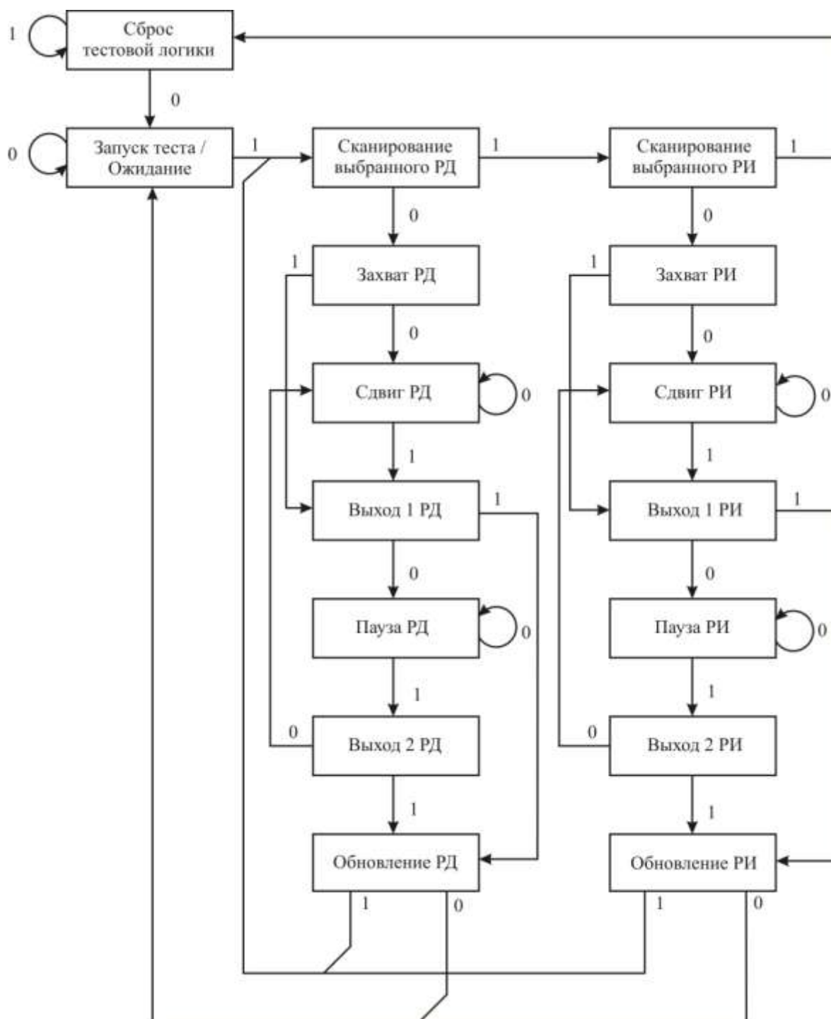
Рисунок 3.122 – Диаграмма состояний TAP-контроллера
