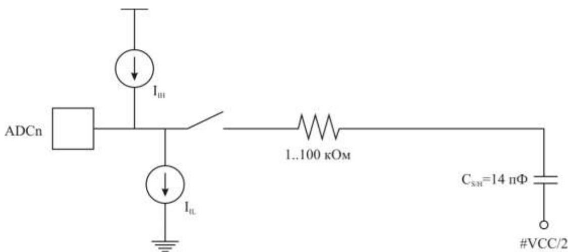
Рисунок 3.114 – Схема аналогового входа
