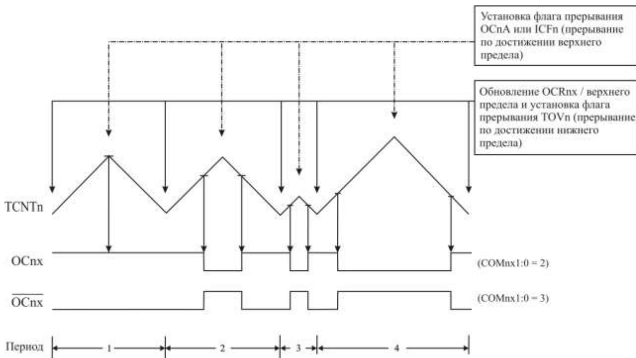
Рисунок 3.55 – Временная диаграмма для режима широтно-импульсной модуляции с фазовой и частотной коррекцией
