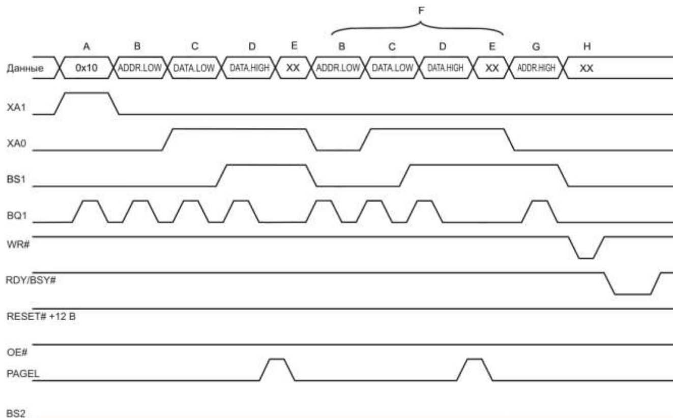
Рисунок 3.138 – Программирование форм сигналов для памяти программ
