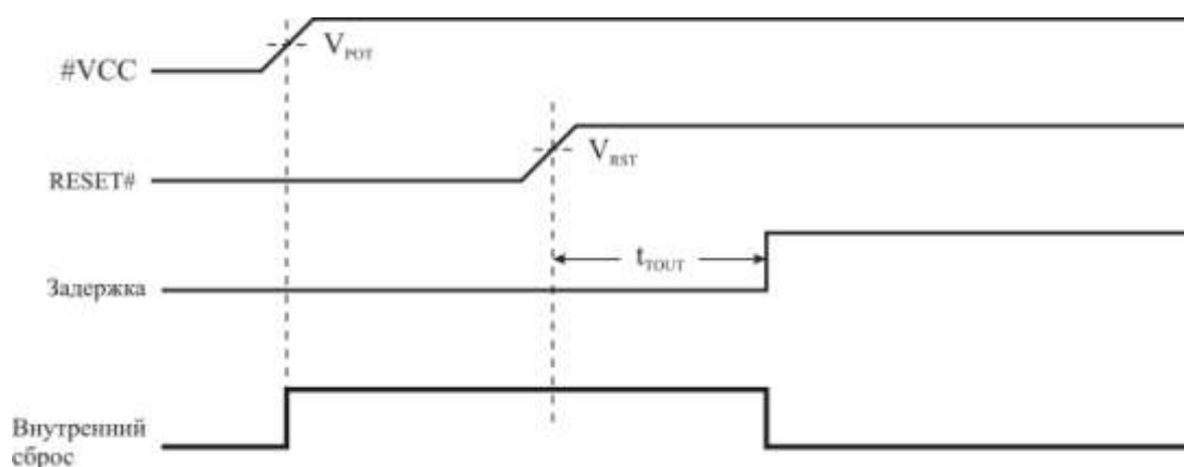
Рисунок 3.25 – Запуск микроконтроллера, RESET# управляется внешне
