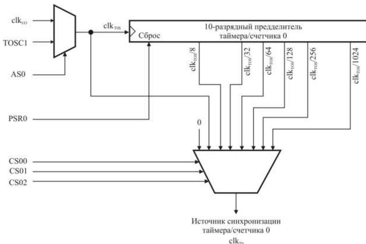
Рисунок 3.46 – Предделитель таймера/счетчика 0
