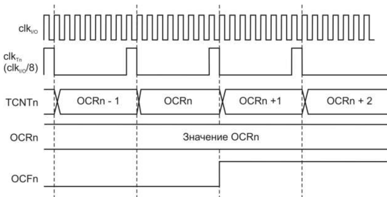
Рисунок 3.44 – Временная диаграмма таймера/счетчика, установка флага OCF0, с делением ( f_{clk\_I/O}/8 )
