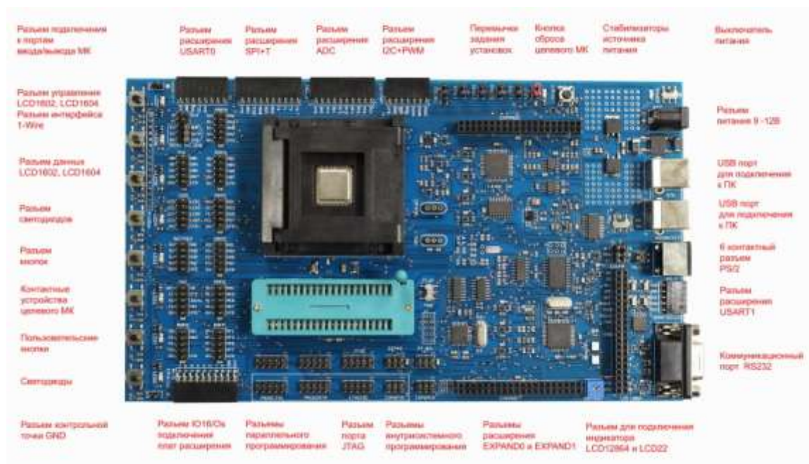
Рисунок 6.1 – Отладочная плата КФДЛ.301411.243
