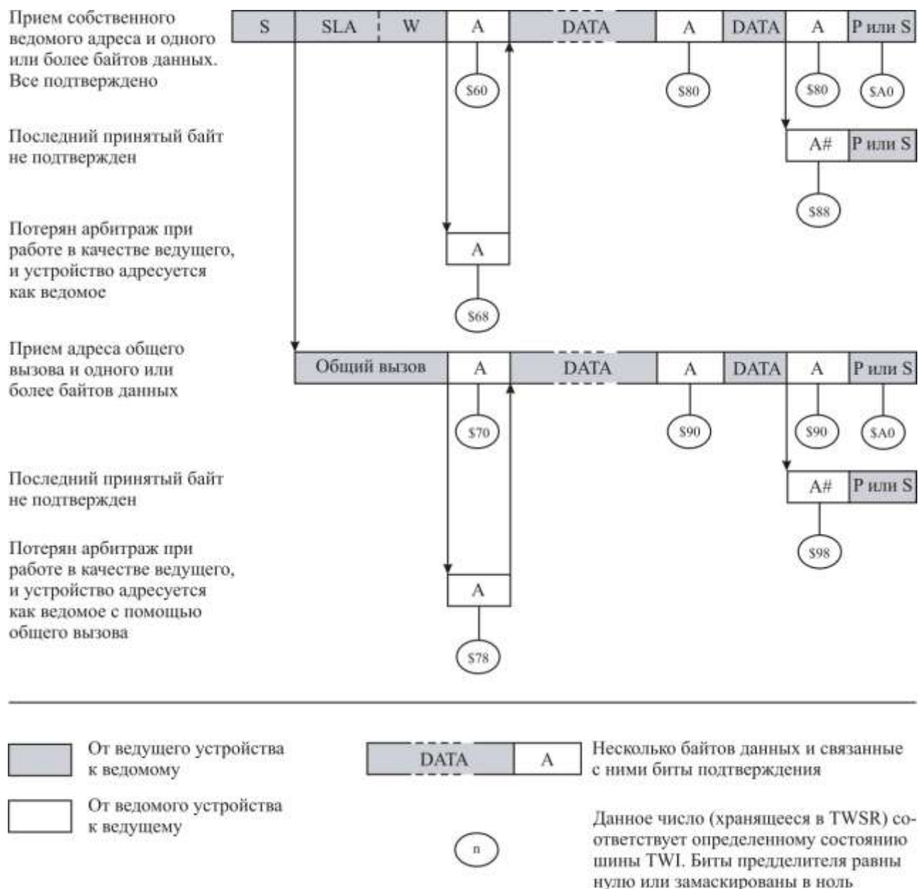
Рисунок 3.102 – Форматы и состояния в режиме ведомого приемника
