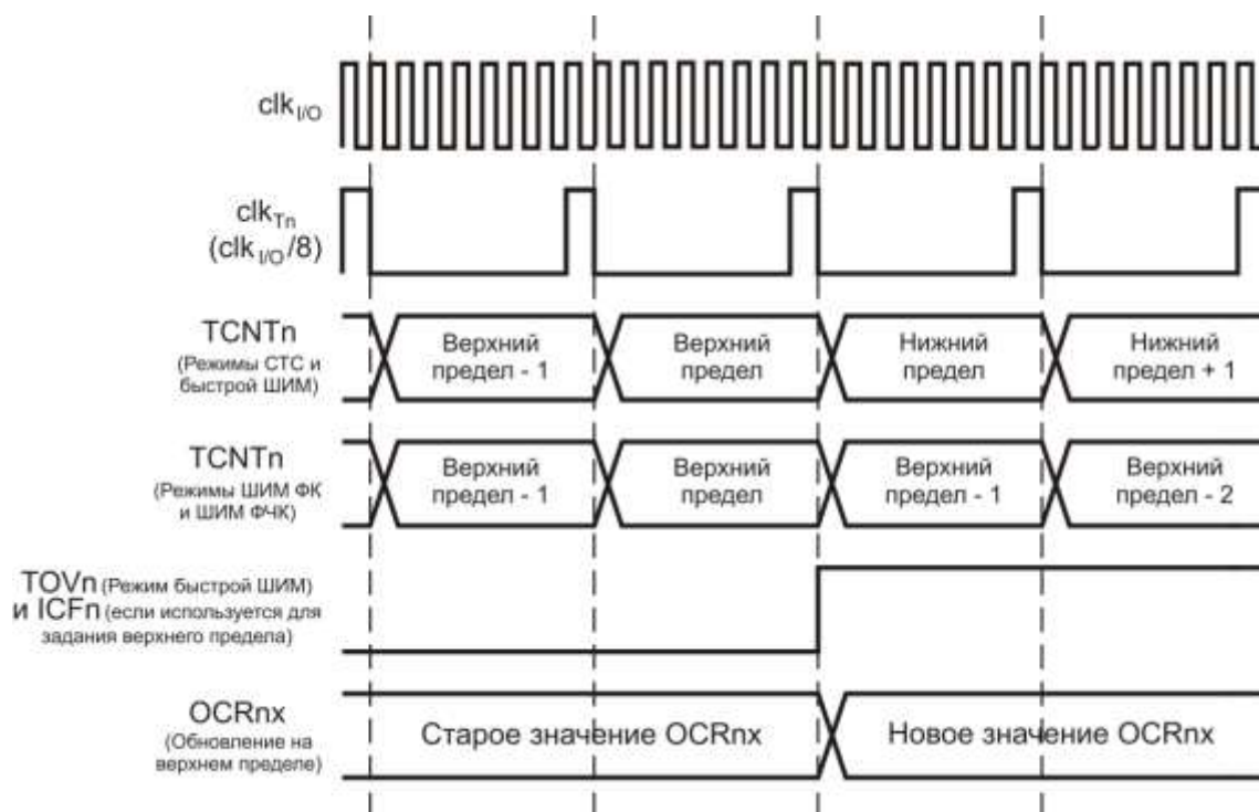
Рисунок 3.59 - Временная диаграмма таймера/счетчика с предделением ( f_{clk\_I/O}/8 )
