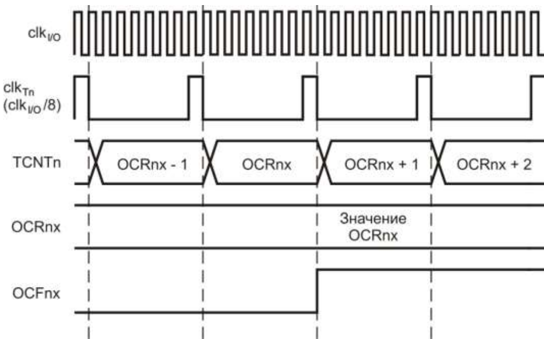
Рисунок 3.57 – Временная диаграмма таймера/счетчика с установкой флага OCFnx и предделением ( f_{clk\_I/O}/8 )
