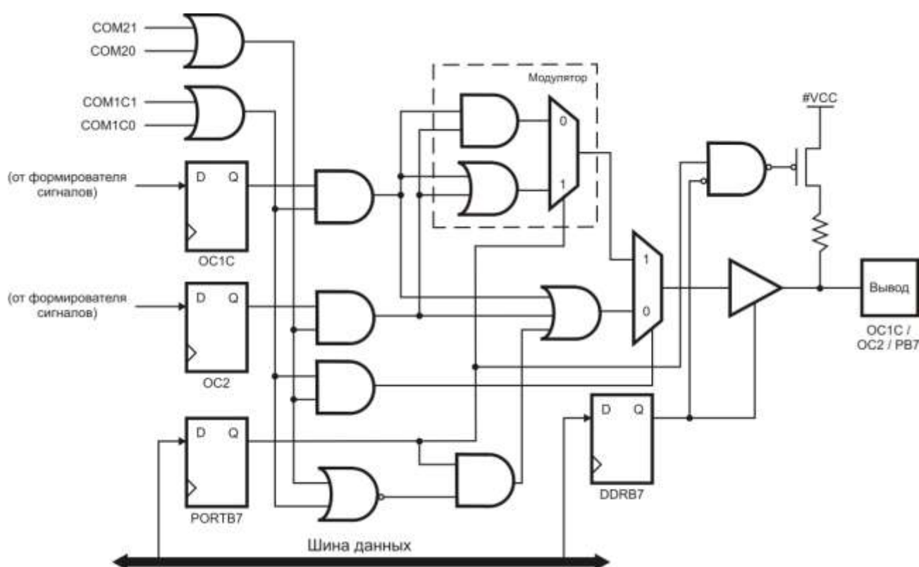
Рисунок 3.74 – Эквивалентная функциональная схема модулятора сравнения
