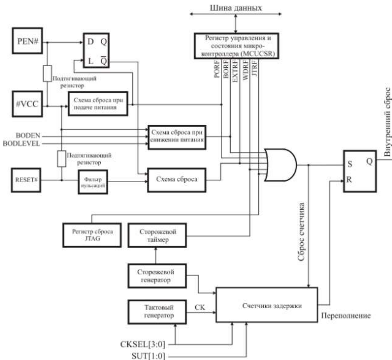
Рисунок 3.23 – Логика сброса
