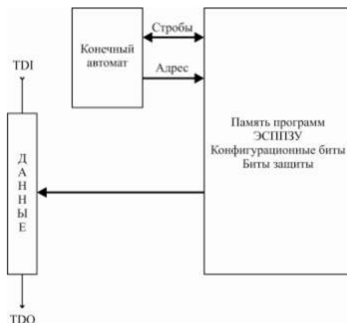
Рисунок 3.152 – Виртуальный регистр чтения страницы памяти программ
