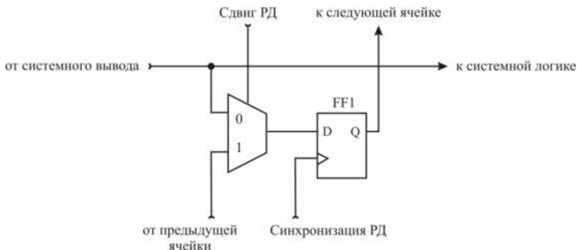
Рисунок 3.128 – Ячейка, предназначенная только для наблюдения
