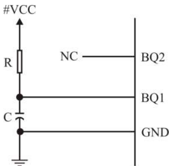
Рисунок 3.21 – Схема подключения внешней задающей RC-цепи
