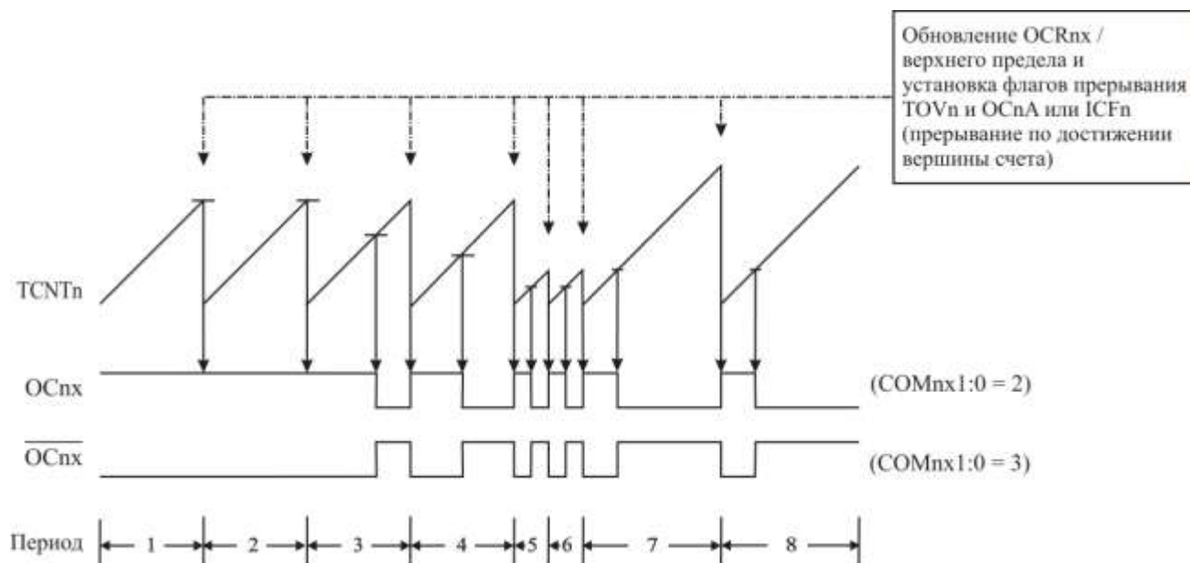
Рисунок 3.53 – Временная диаграмма для режима быстрой ШИМ
