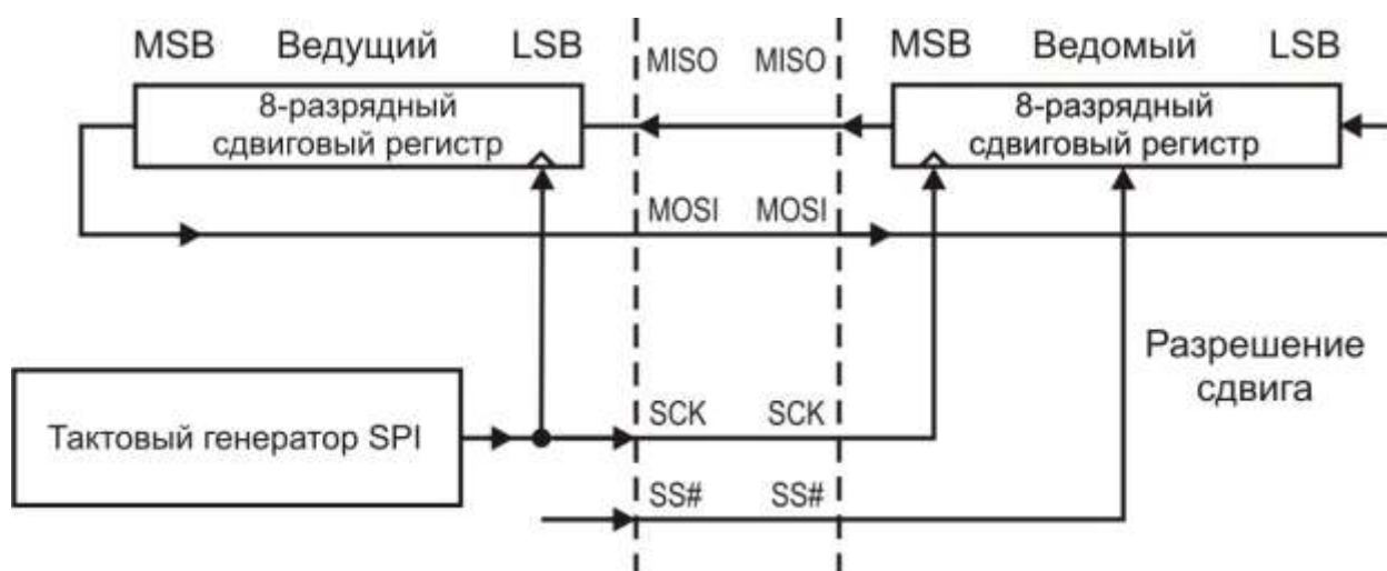
Рисунок 3.77 – Внутреннее соединение ведущего и ведомого SPI
