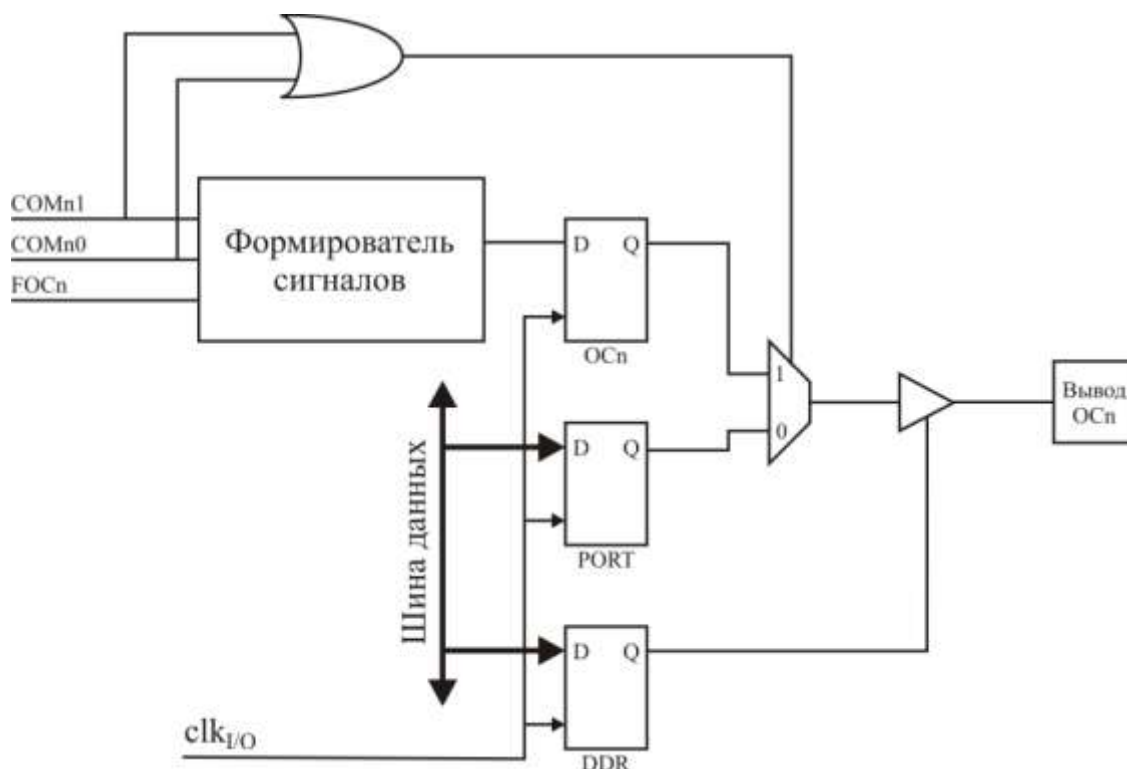
Рисунок 3.65 – Схема блока формирования выходного сигнала
