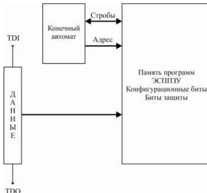
Рисунок 3.151 – Виртуальный регистр загрузки страницы памяти программ
