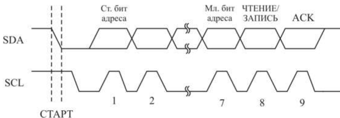
Рисунок 3.90 – Формат адресного пакета
