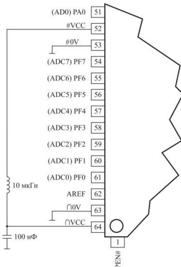
Рисунок 3.115 – Подключение питания АЦП
