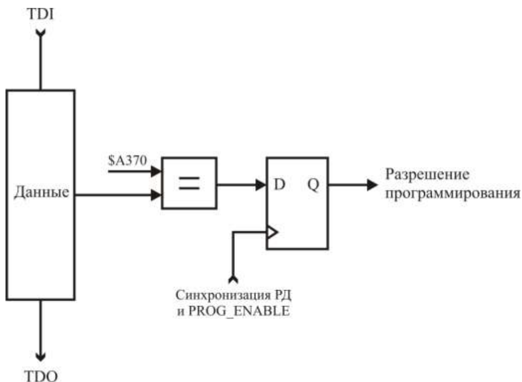
Рисунок 3.148 – Регистр разрешения программирования
