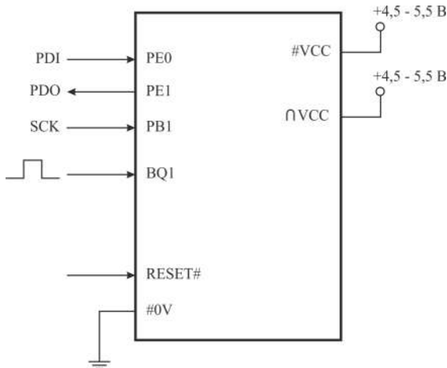
Рисунок 3.145 – Последовательное программирование и проверка
