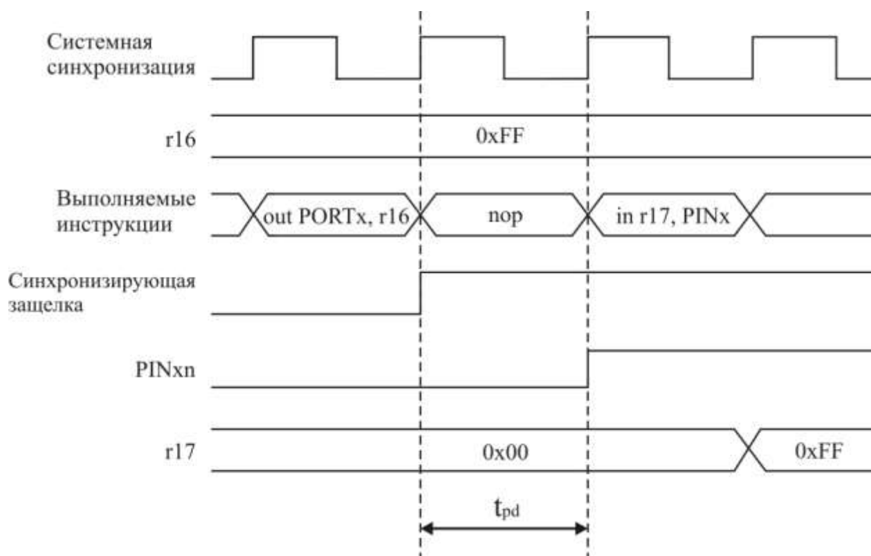
Рисунок 3.33 – Синхронизация при считывании программно установленного состояния вывода
