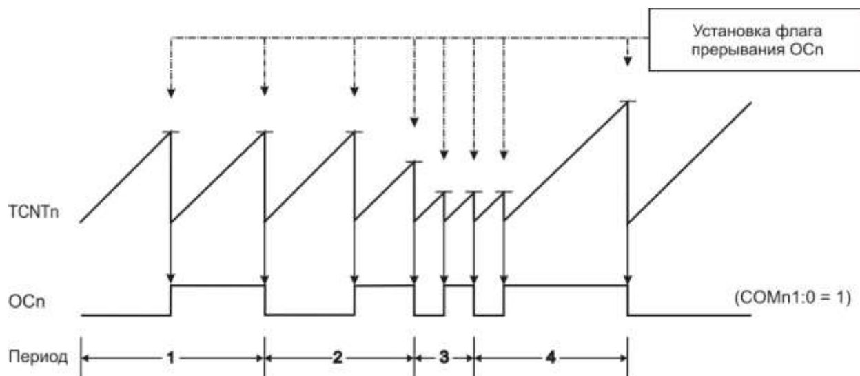
Рисунок 3.39 – Временная диаграмма для режима CTC
