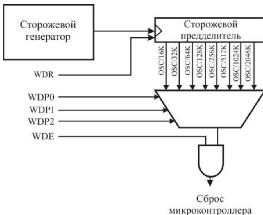
Рисунок 3.29 – Сторожевой таймер
