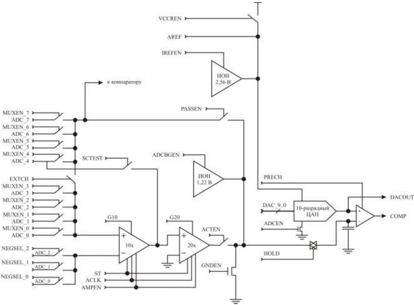
Рисунок 3.132 – Аналого-цифровой преобразователь
