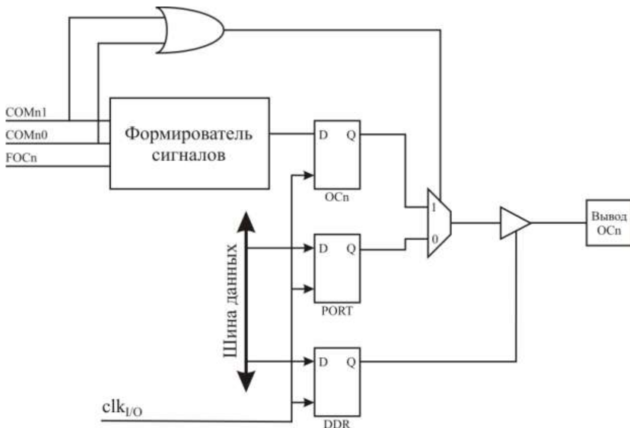
Рисунок 3.38 – Схема блока формирования выходного сигнала
