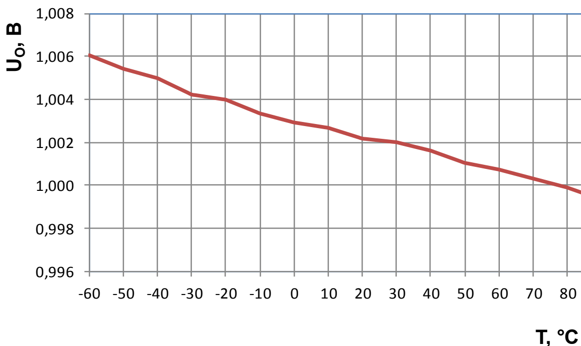
Рисунок 5 – Зависимость минимального выходного напряжения U_o микросхемы 1309ЕР1Т от температуры корпуса при U_i = 2 В, I_o = 10 мА
