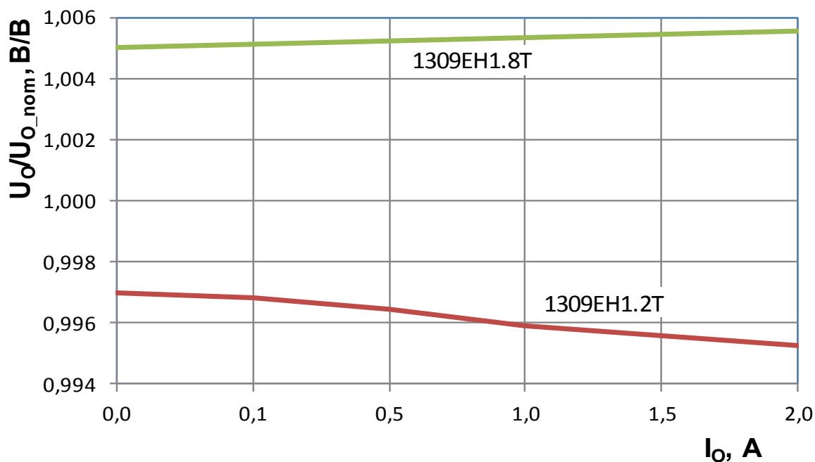
Рисунок 8 – Зависимость выходного напряжения U_o (приведенного к выходному напряжению номинальному U_{o\_nom} ) от тока нагрузки при U_i = 2,8 В для 1309ЕН1.2Т и U_i = 2,6 В для 1309ЕН1.8Т, T = 25 °С
