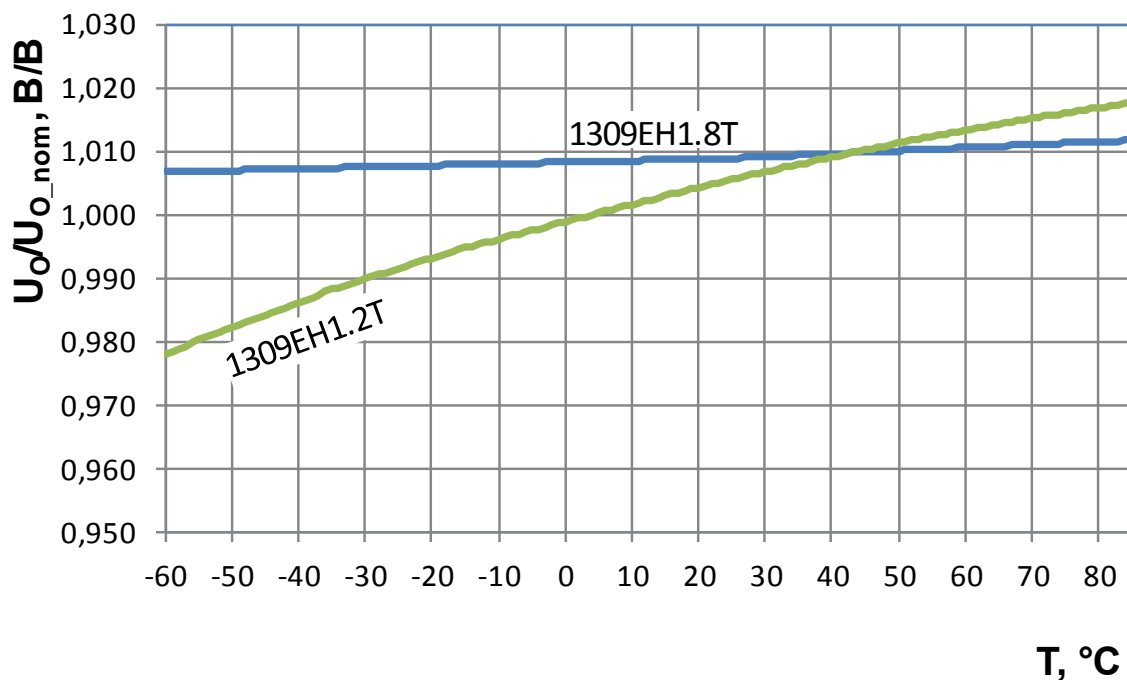
Рисунок 4 – Зависимость выходного напряжения U_o (приведенного к выходному напряжению номинальному U_{o\_nom} ) от температуры корпуса при U_i = U_{i\_min} В, I_o = 10 мА
