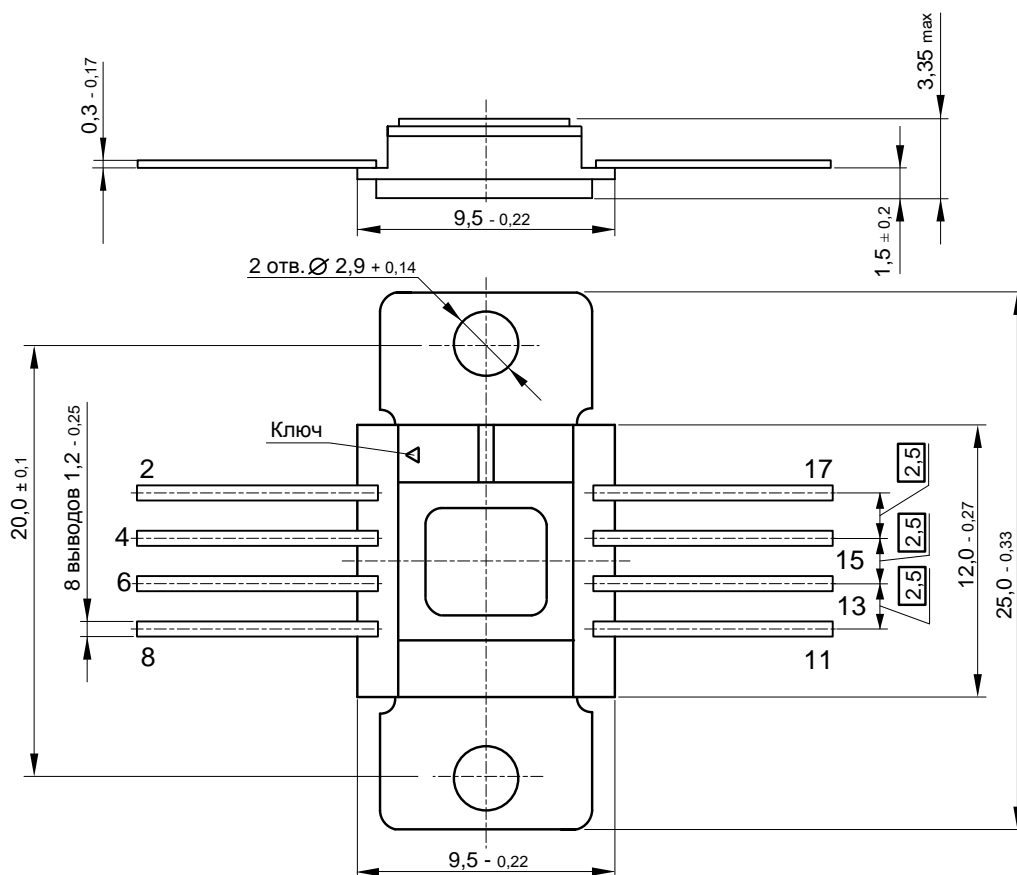
Рисунок 20 – Корпус 4116.8-3
