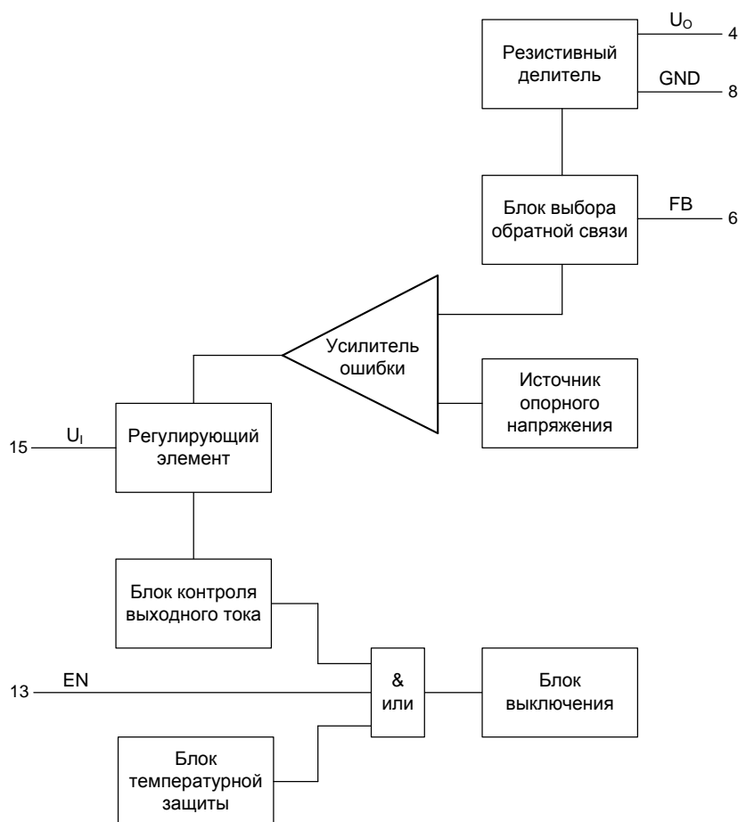
Рисунок 1 – Структурная блок-схема микросхем
