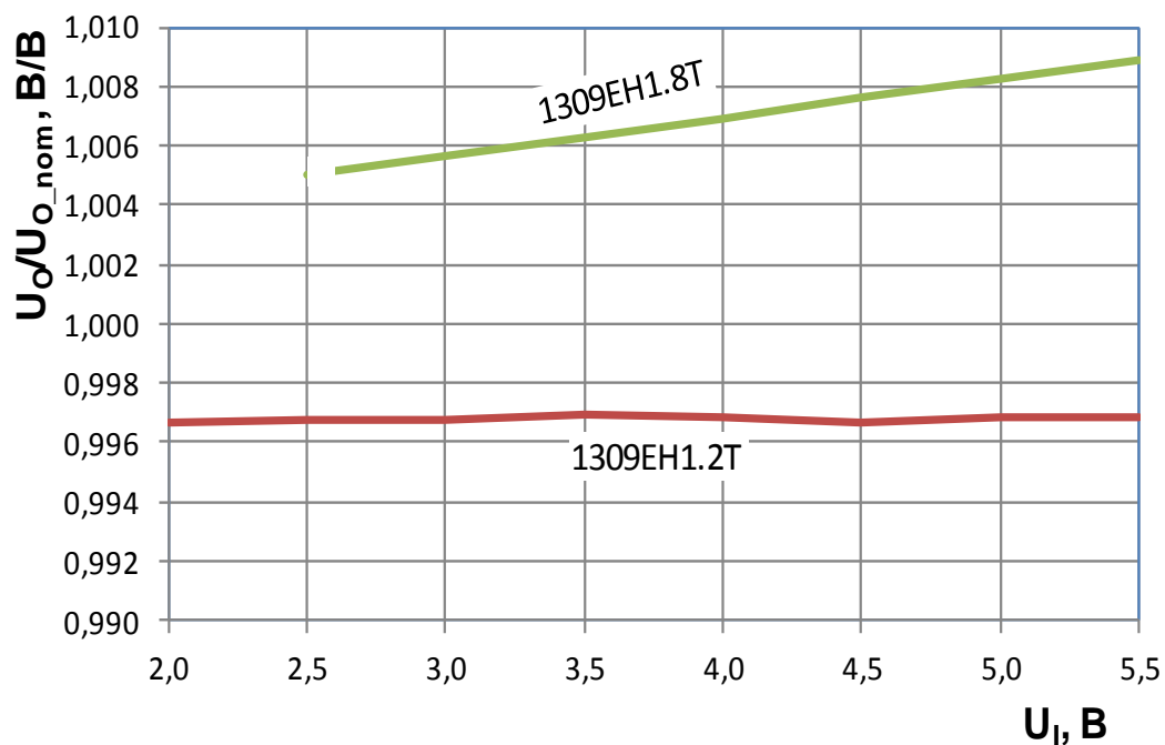
Рисунок 6 – Зависимость выходного напряжения U_o (приведенного к выходному напряжению номинальному U_{o\_nom} ) от входного напряжения при I_o = 100 мА, T = 25 °С
