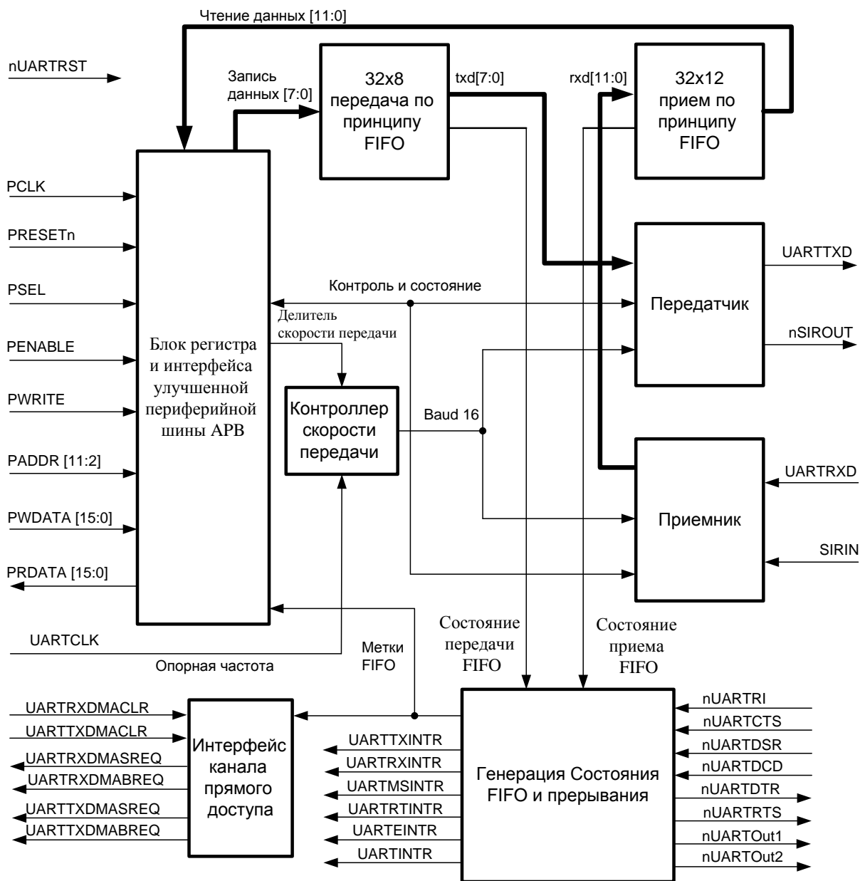
Рисунок 77 – Блок-схема универсального асинхронного приёмопередатчика (УАП)
