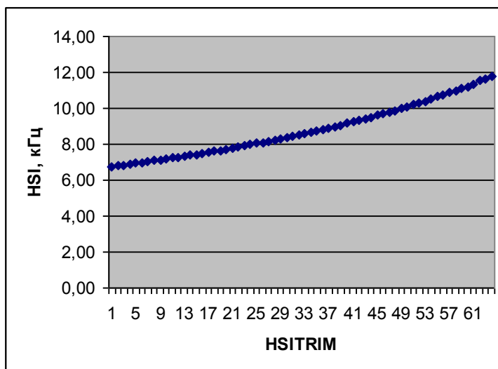
Рисунок 25 – Зависимость частоты HSI от значения HSITRIM
