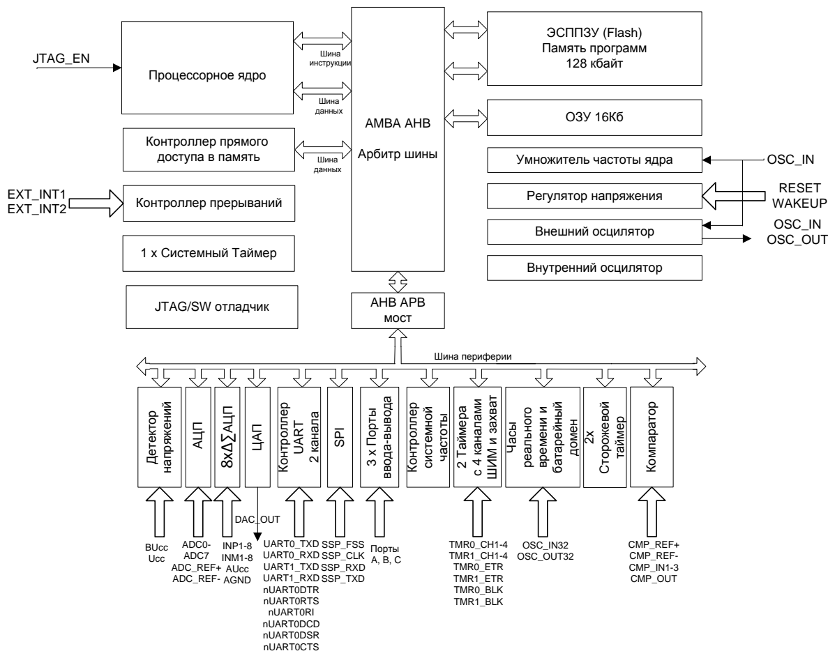
Рисунок 1 – Структурная схема
