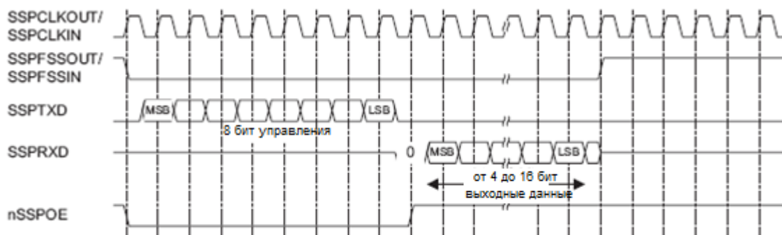
Рисунок 70 – Формат синхронного обмена протокола Microwire фирмы National Semiconductor (одиночный обмен)
