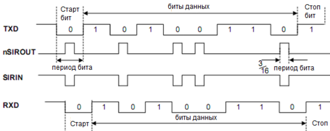
Рисунок 80 – Модуляция данных IrDA
