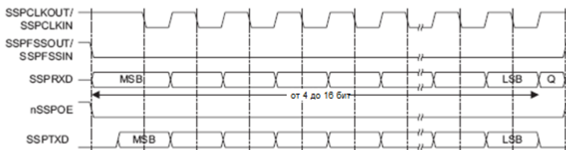
Рисунок 67 – Формат синхронного обмена протокола SPI фирмы Motorola, SPO=1, SPH=0 (одиночный обмен)
