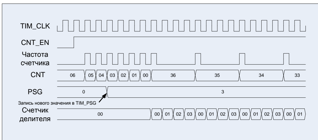
Рисунок 34 – Диаграммы работы счетчика: счет вниз (CNT_MODE = 00, EVENT_SEL = 0000, DIR = 1)
