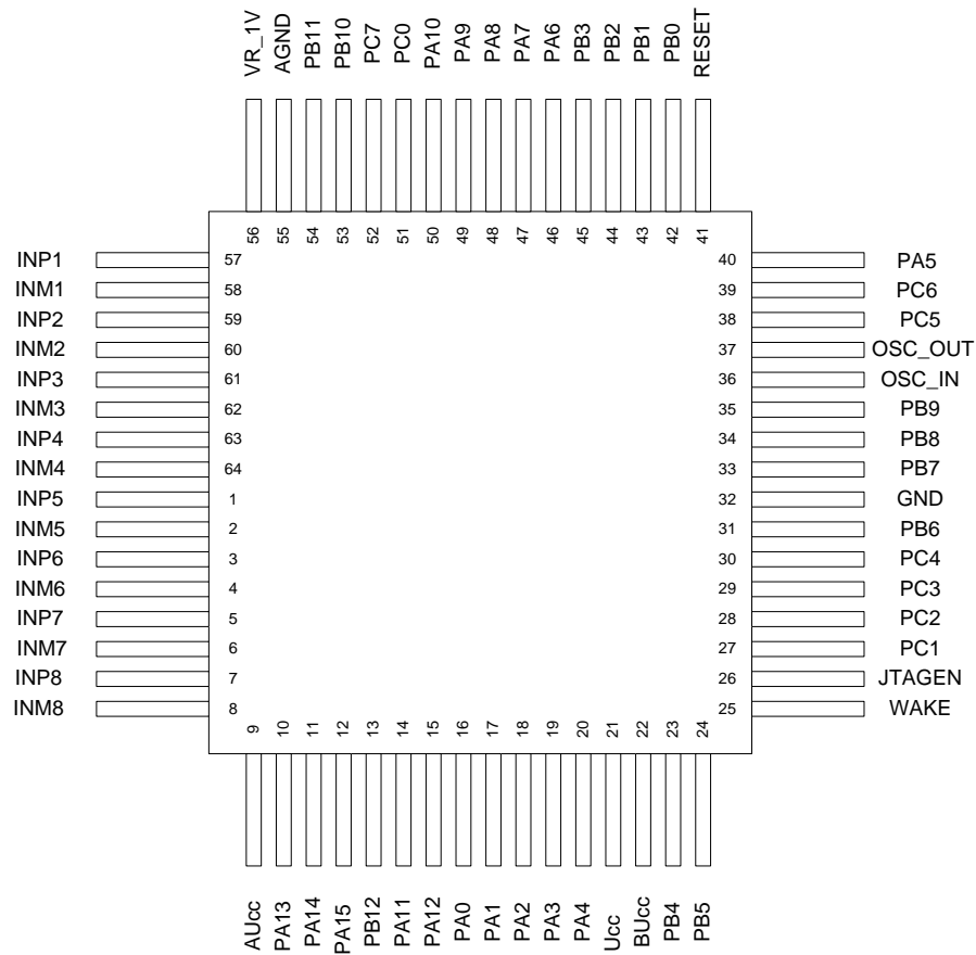
Рисунок 2 – 64-х выводной металлокерамический корпус Н18.64-1В
