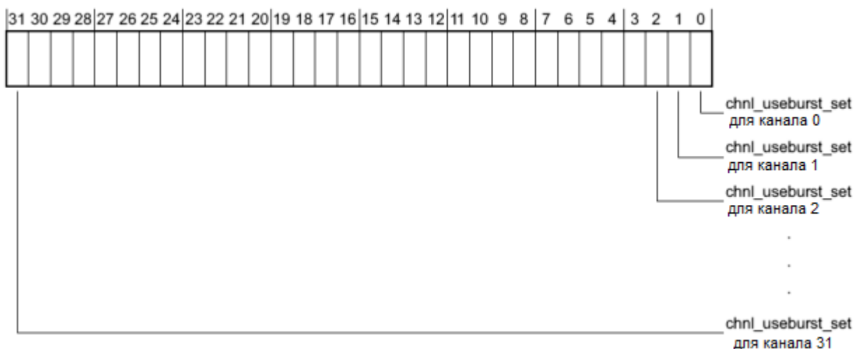
Рисунок 105 – Наименование разрядов регистра chnl_useburst_set
