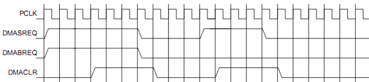
Рисунок 83 – Временные диаграммы одноэлементного и блочного запросов DMA
