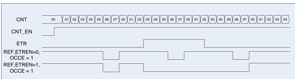
Рисунок 49 – Диаграмма работы схемы в режиме ШИМ, CCR1_EN = 0
