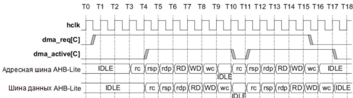
Рисунок 88 – Диаграмма работы при получении от периферийного блока запроса на обработку по уровню
