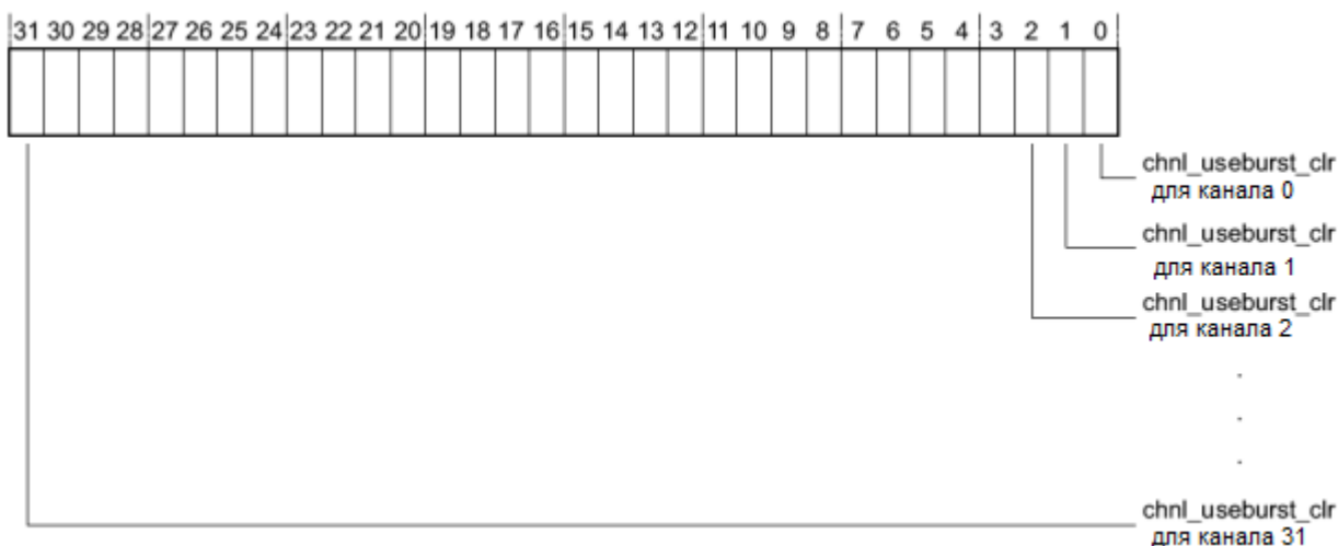
Рисунок 106 – Наименование разрядов регистра chnl_useburst_clr
