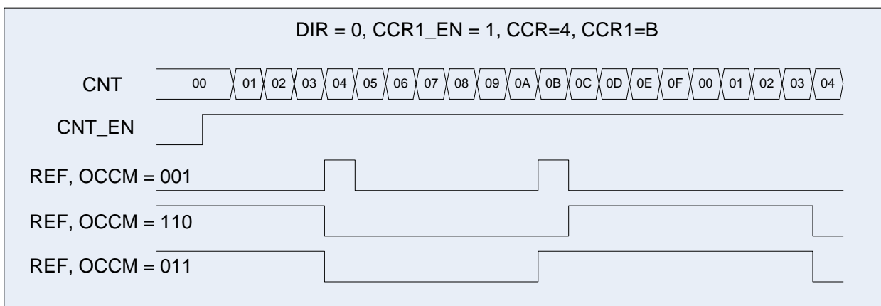
Рисунок 51 – Диаграмма работы схемы в режиме ШИМ, CCR1_EN = 1
