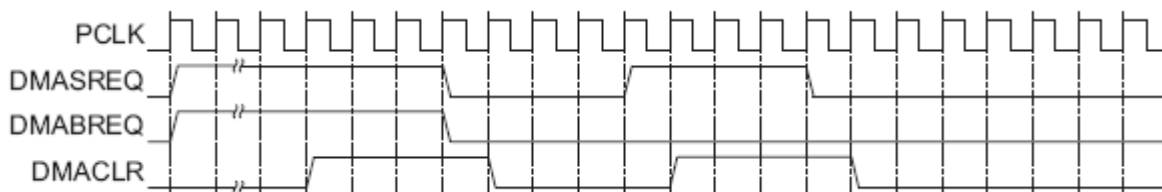
Рисунок 76 – Временные диаграммы обмена в режиме ПДП
