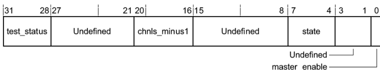
Рисунок 99 – Наименование разрядов регистра dma_status
