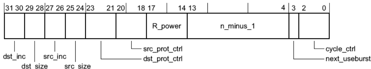
Рисунок 98 – Название разрядов channel_cfg
