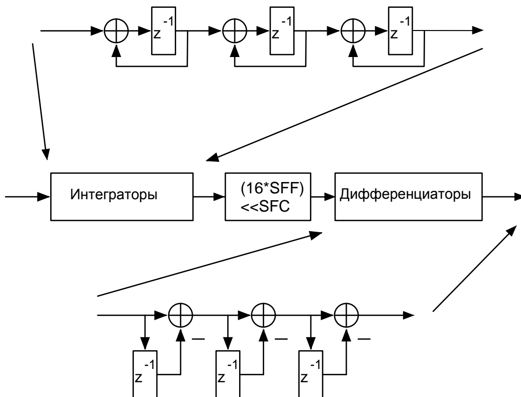
Рисунок 20 – Структурная схема SYNC 3 фильтра
