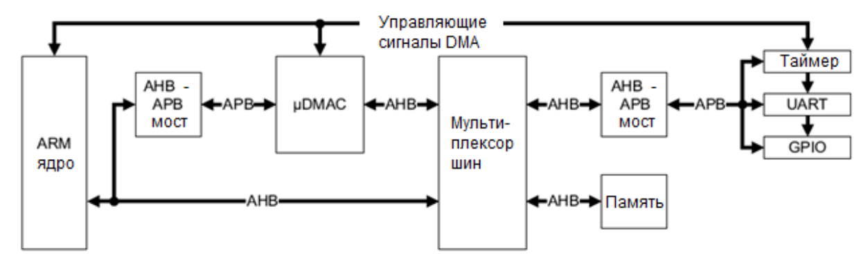
Рисунок 86 – Пример структурной схемы микроконтроллера с использованием контроллера ПДП
