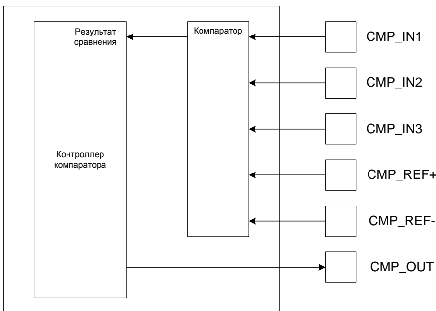
Рисунок 58 – Структура блока компаратора
