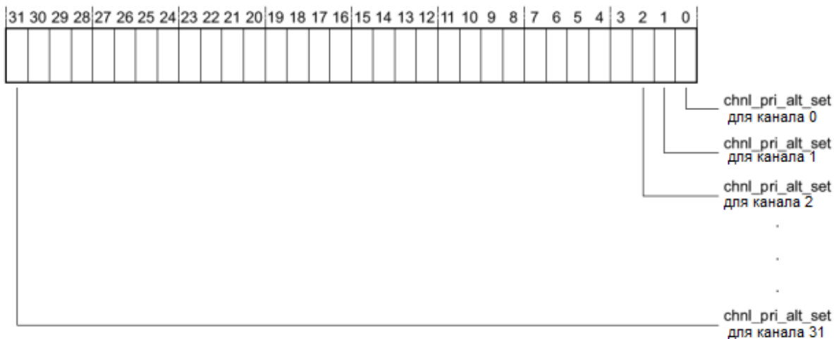
Рисунок 111 – Наименование разрядов регистра chnl_pri_alt_set
