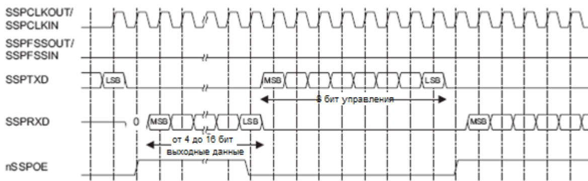
Рисунок 71 – Формат синхронного обмена протокола Microwire фирмы National Semiconductor (непрерывный обмен)
