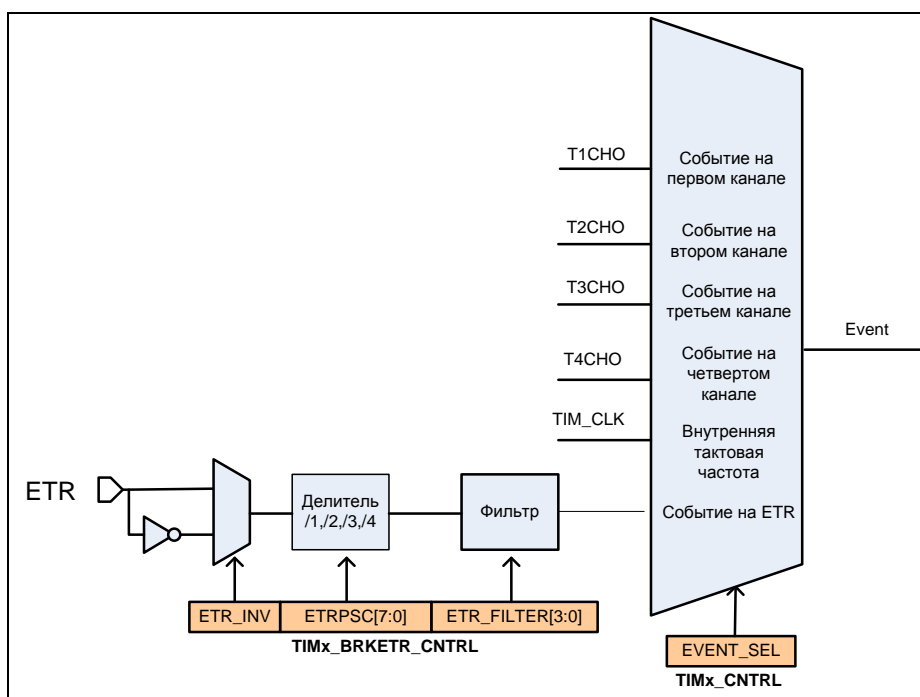
Рисунок 42 – Схема тактирования сигналом со входа ETR
