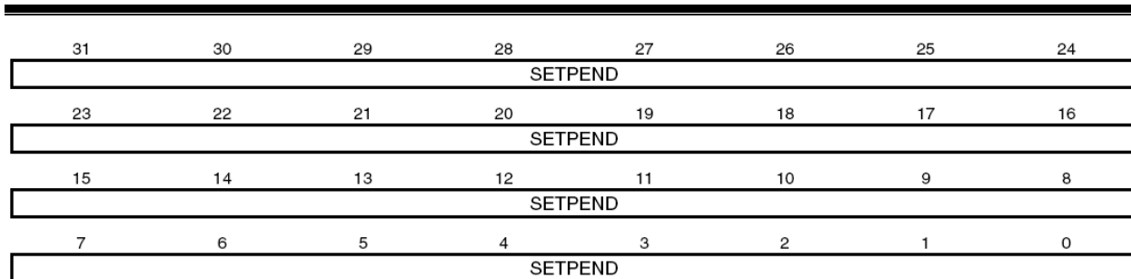
Рисунок 119 – Распределение битов регистра ISPR
