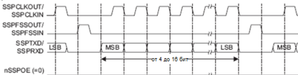
Рисунок 65 – Формат синхронного обмена протокола SPI фирмы Motorola, SPO=0, SPH=0 (непрерывный обмен)
