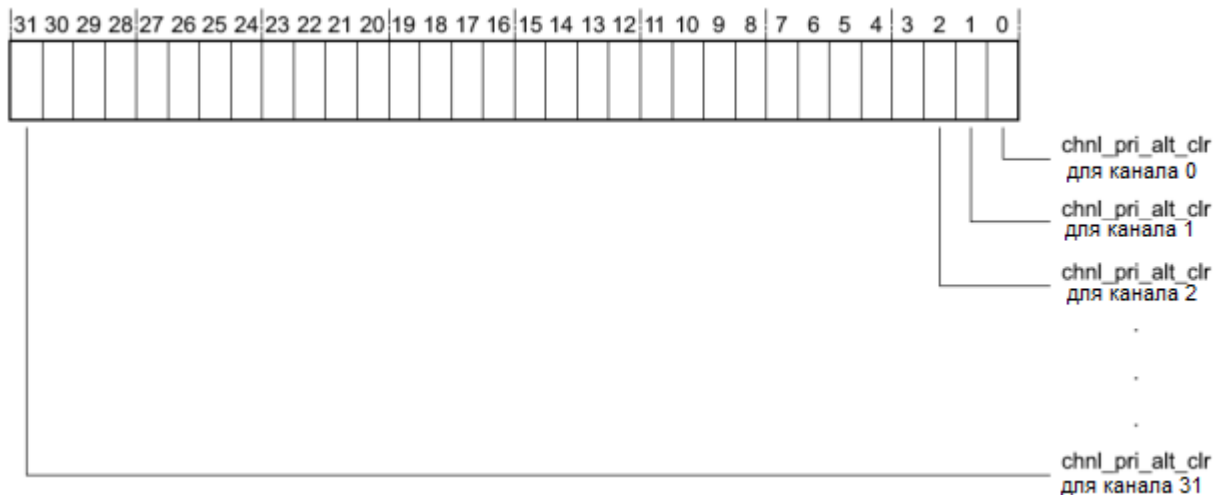
Рисунок 112 – Наименование разрядов регистра chnl_pri_alt_clr
