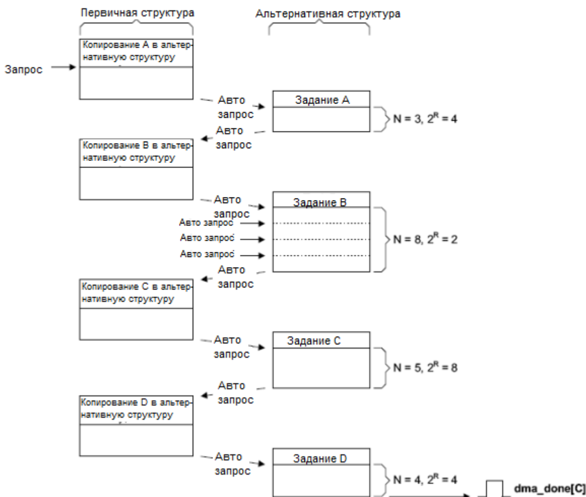
Рисунок 94 – Пример функционирования контроллера в режиме работы с памятью «исполнение с изменением конфигурации».
