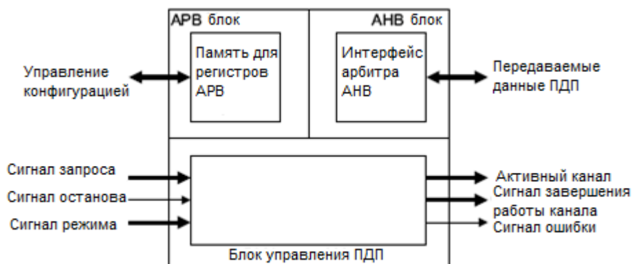
Рисунок 84 – Структурная схема контроллера DMA
