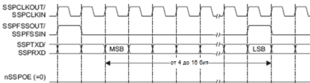
Рисунок 63 – Формат синхронного обмена протокола SSI фирмы Texas Instruments (непрерывный обмен)
