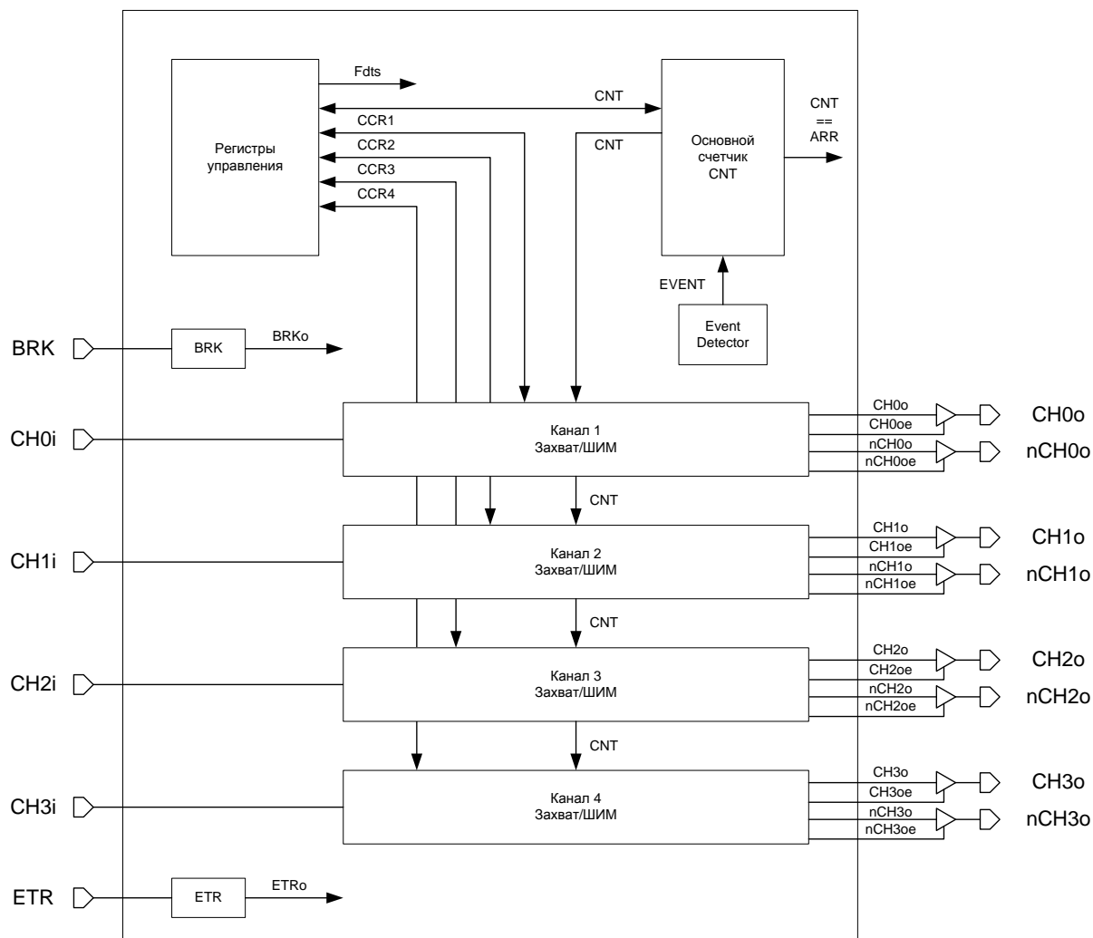
Рисунок 27 – Структурная схема таймера
