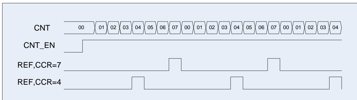
Рисунок 47 – Диаграмма работы схемы в режиме ШИМ, CCR1_EN=0
