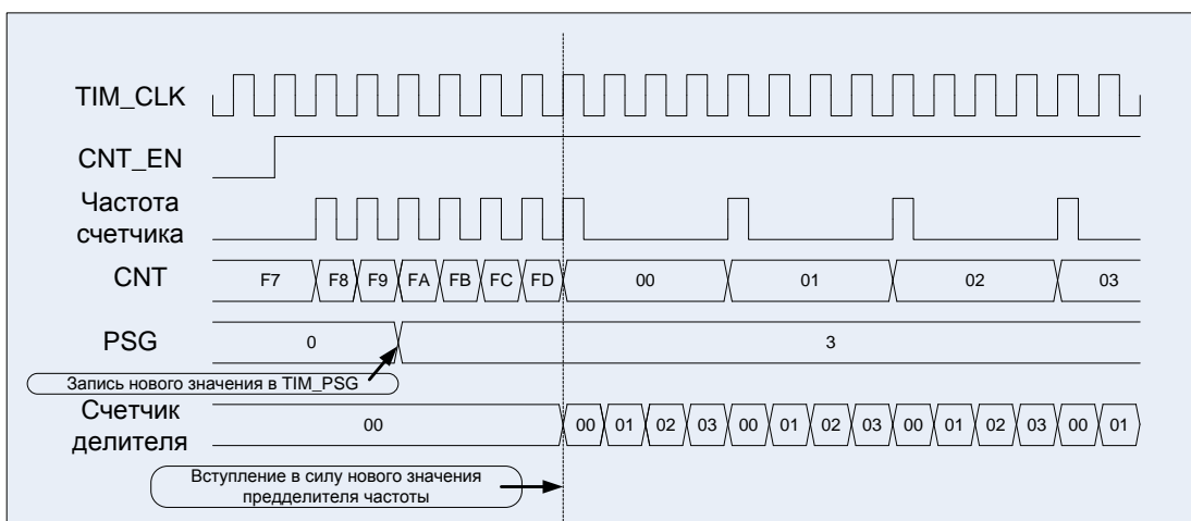
Рисунок 33 – Диаграммы работы счетчика: счет вверх (CNT_MODE = 00, EVENT_SEL = 0000, DIR = 0)
