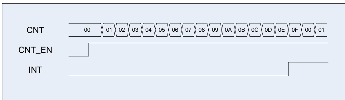
Рисунок 52 – Режим обычного счетчика
