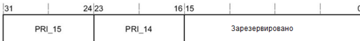
Рисунок 128 – Назначение разрядов регистра
