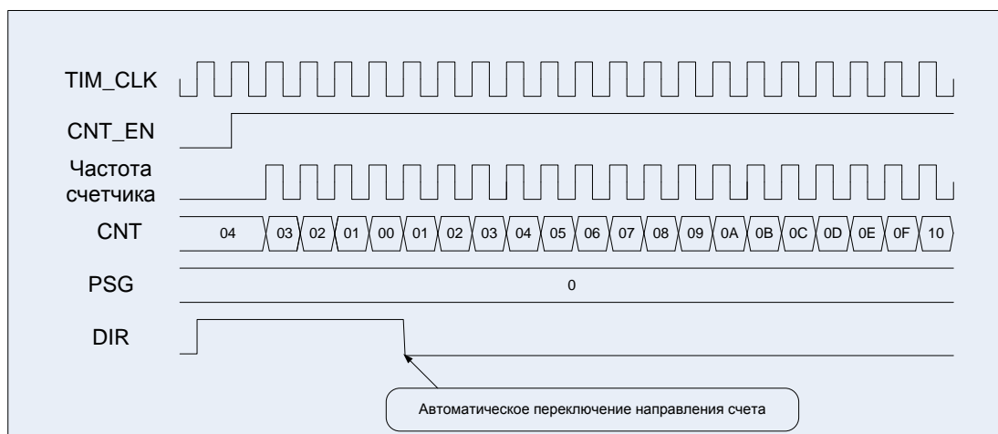
Рисунок 31 – Диаграммы работы таймера, счет вверх/вниз, сначала вниз
