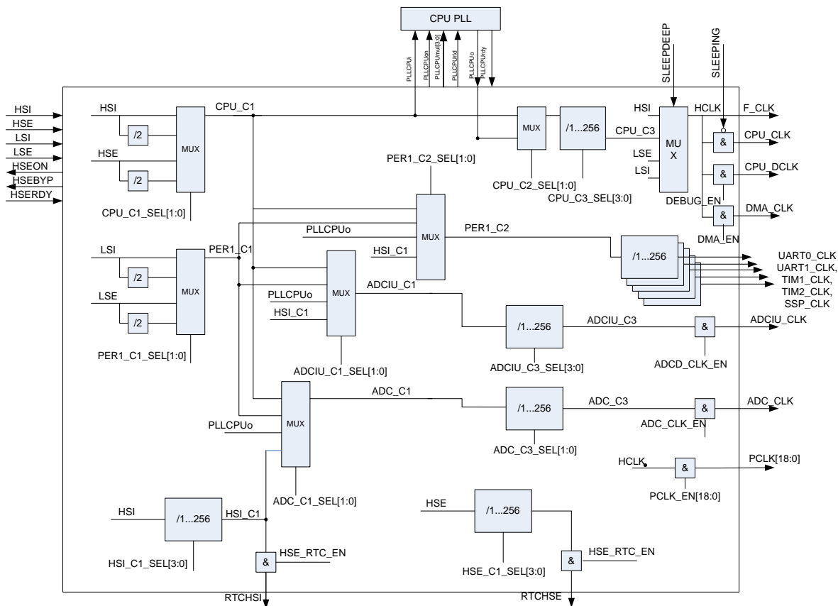
Рисунок 22 – Структурная блок – схема формирования тактовой частоты
