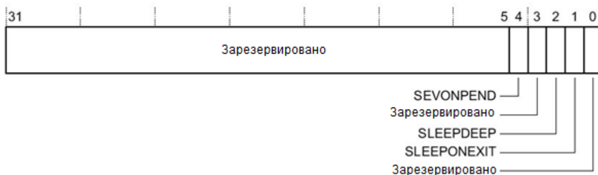
Рисунок 125 – Назначение разрядов регистра SCR
