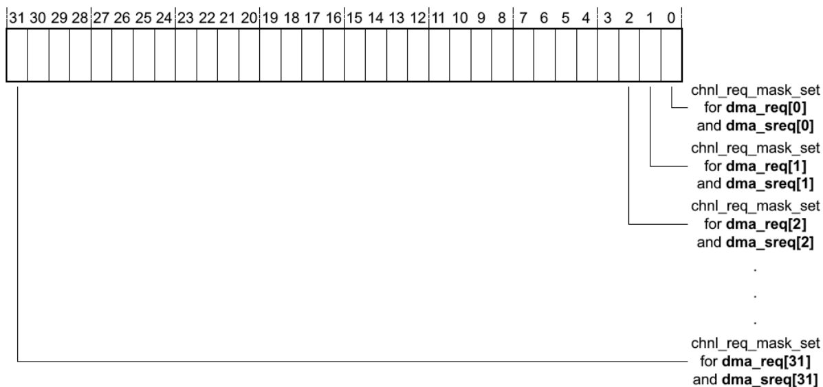
Рисунок 107 – Наименование разрядов регистра chnl_req_mask_set
