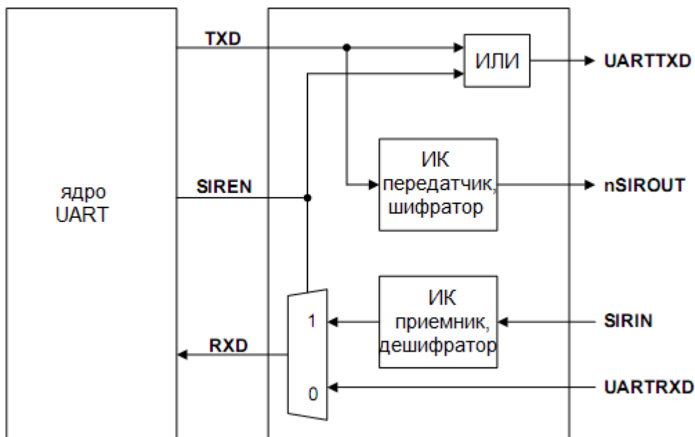
Рисунок 78 – Структурная схема кодека
