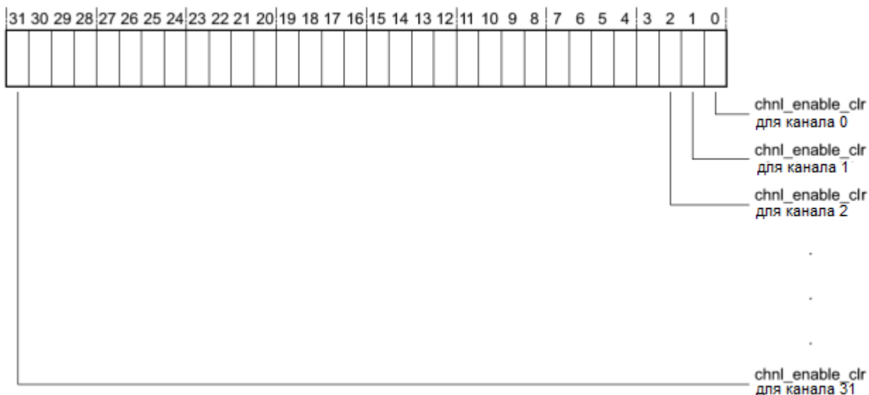
Рисунок 110 – Наименование разрядов регистра chnl_enable_clr
