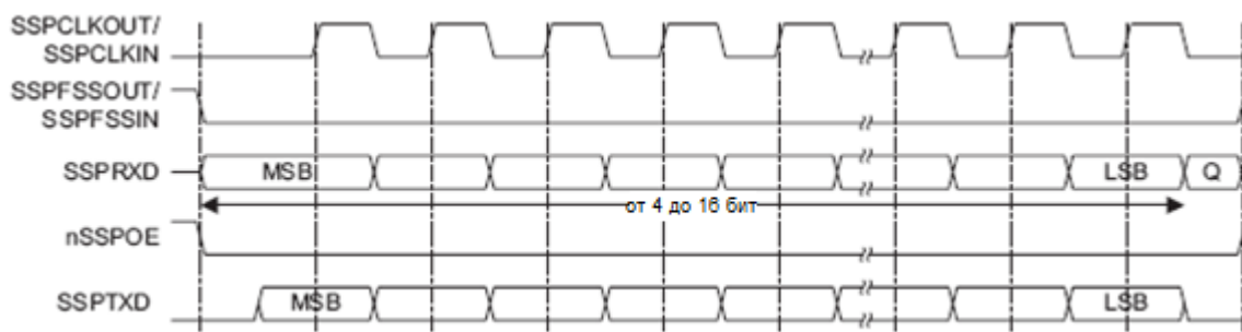
Рисунок 64 – Формат синхронного обмена протокола SPI фирмы Motorola, SPO=0, SPH=0 (одиночный обмен)
