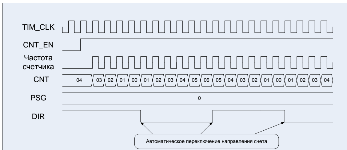
Рисунок 35 – Диаграммы работы счетчика: счет вниз/вверх (CNT_MODE = 01, EVENT_SEL = 0000, DIR = 1)
