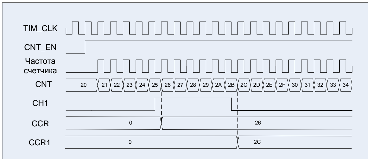
Рисунок 45 – Диаграмма захвата события со входа первого канала
