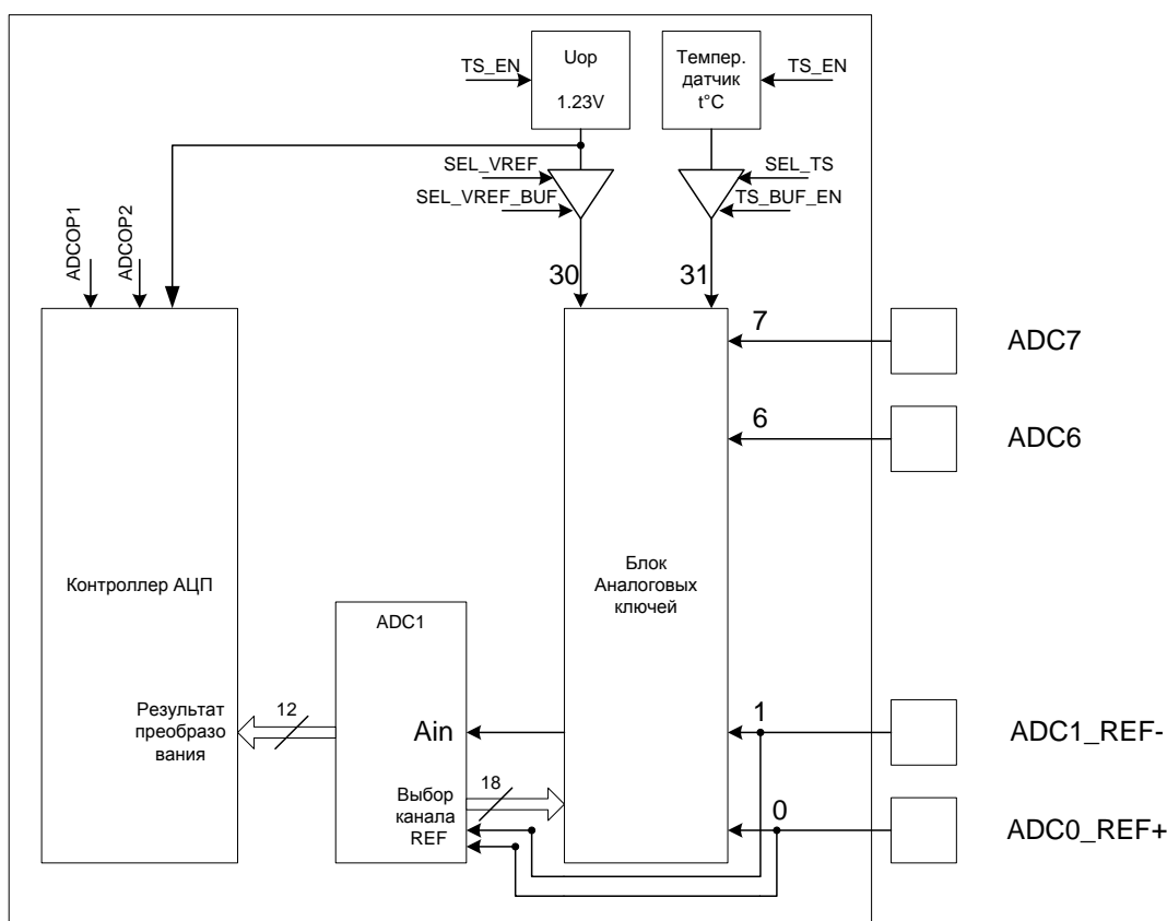
Рисунок 55 – Структурная схема контроллера АЦП
