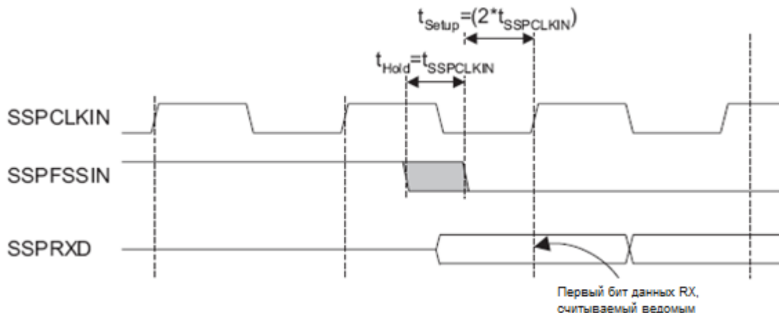
Рисунок 72 – Формат кадра Microwire, требования к времени установки и удержания сигнала SSPFSSIN
