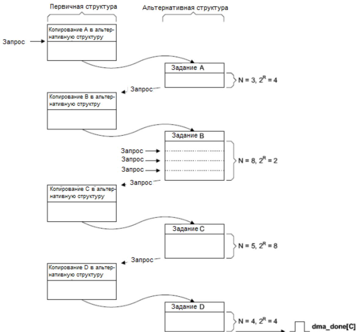
Рисунок 95 – Пример функционирования контроллера в режиме работы с периферией «исполнение с изменением конфигурации»
