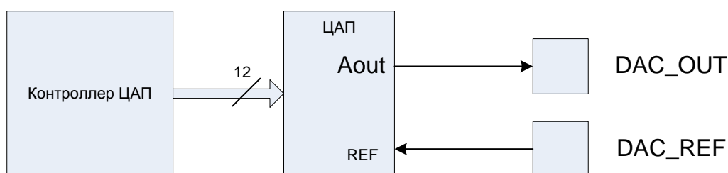
Рисунок 57 – Структурная схема контроллера ЦАП
