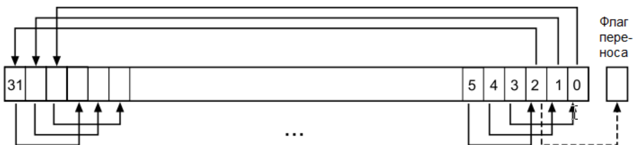
Рисунок 19 – Инструкция ROR # 3
