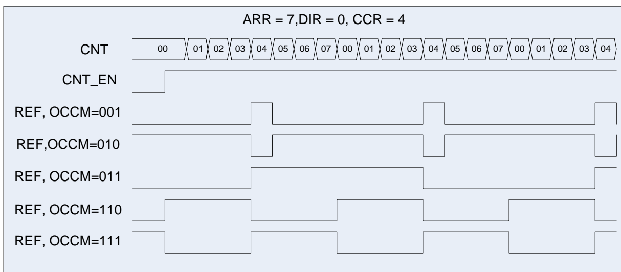
Рисунок 48 – Диаграмма работы схемы в режиме ШИМ, CCR1_EN=0
