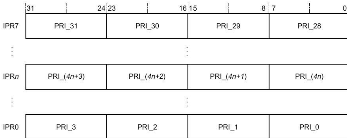
Рисунок 121 – Назначение бит
