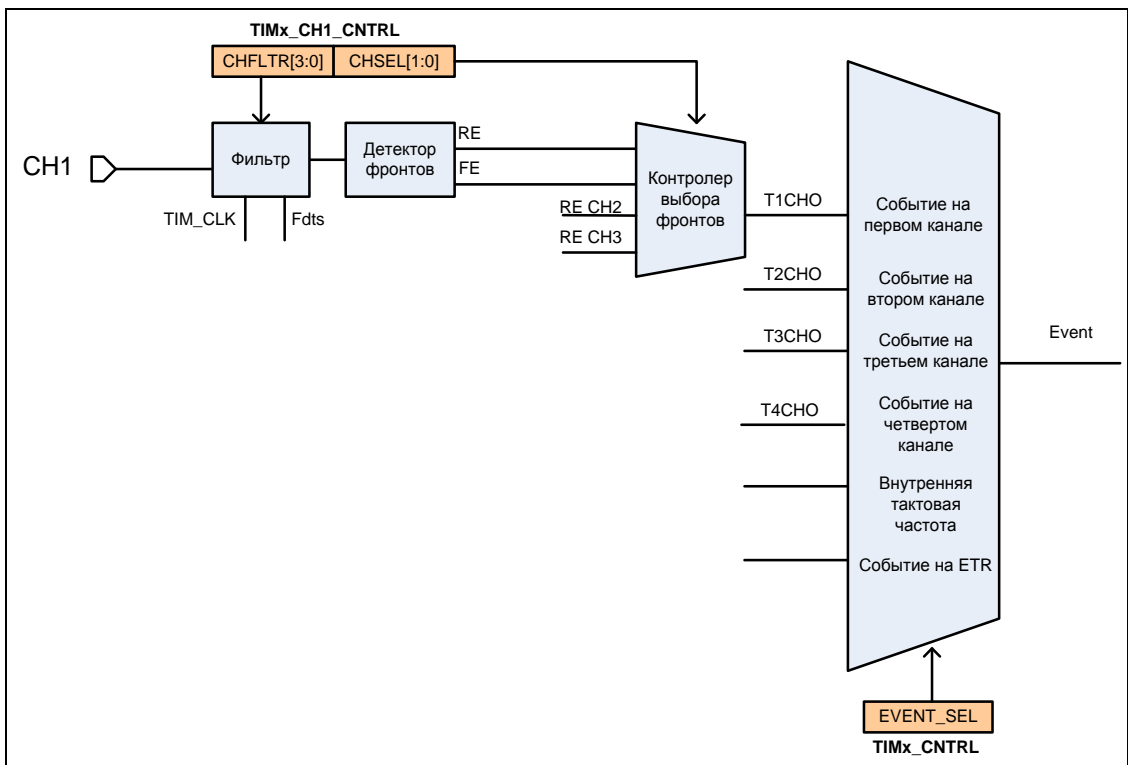
Рисунок 39 – Тактирование с входа первого канала
