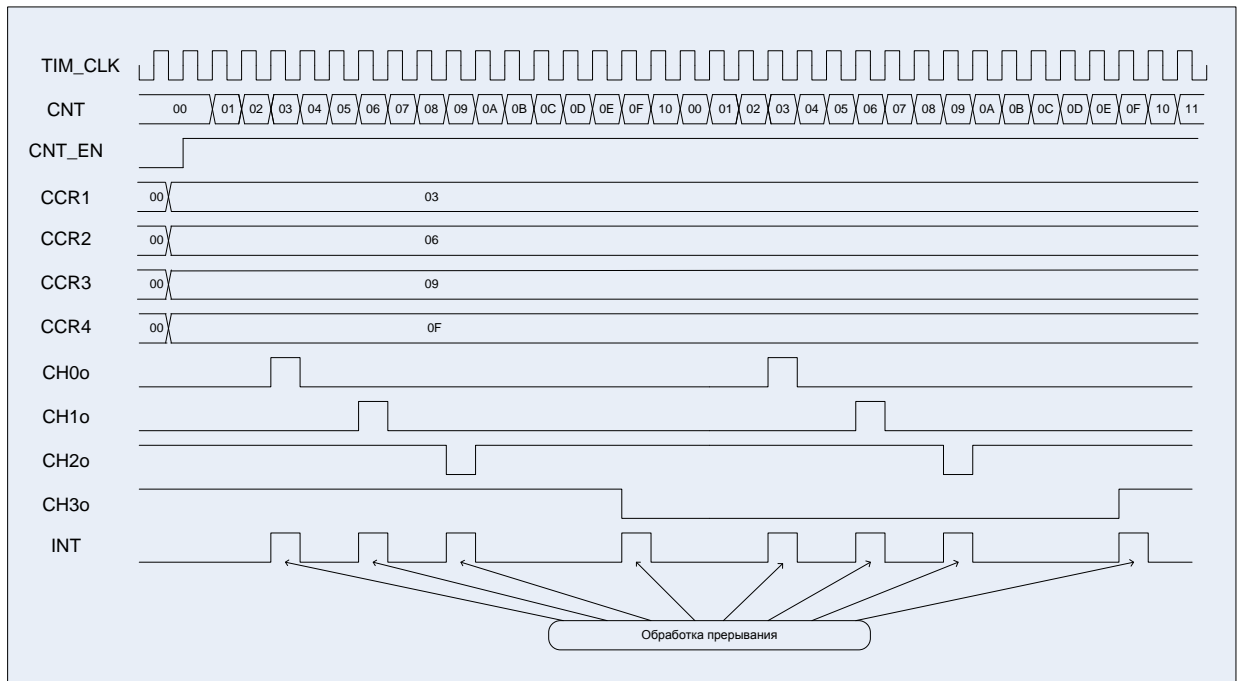
Рисунок 54 – Диаграммы примера работы в режиме ШИМ
