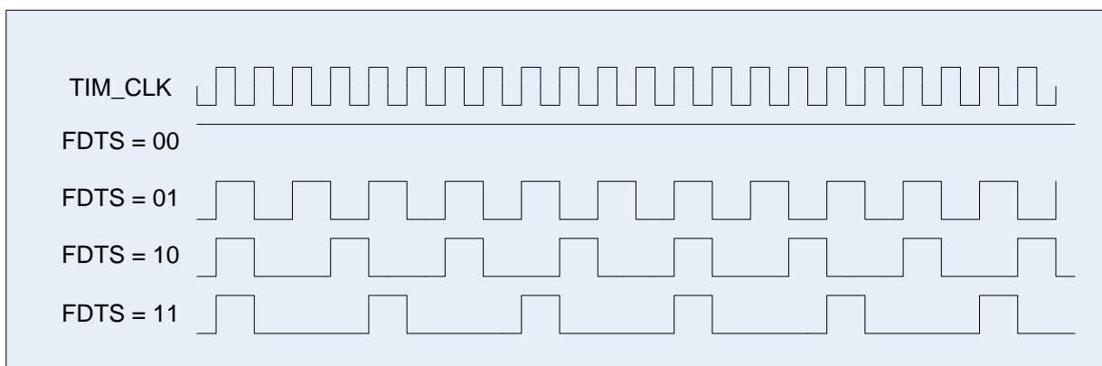
Рисунок 38 – Диаграммы возможных частот семплирования данных (FDS)
