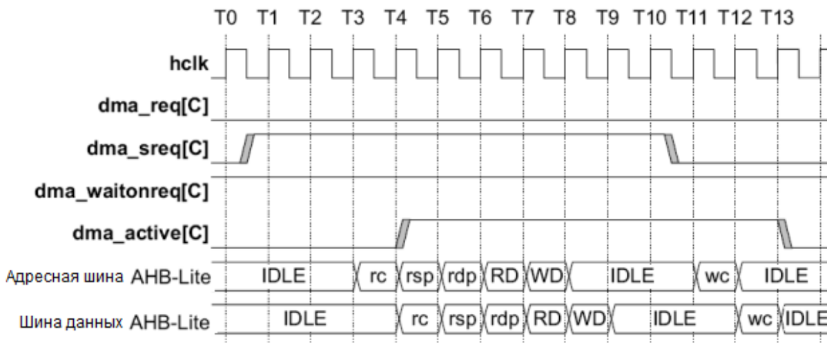
Рисунок 91 – Диаграмма работы контроллера ПДП при использовании периферией dma_waitonreq совместно с dma_sreq
