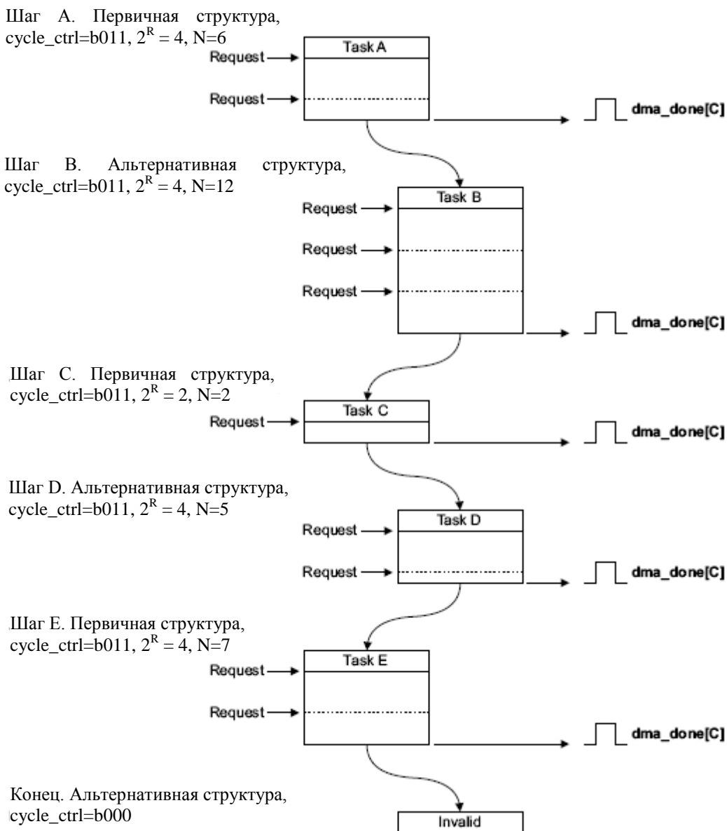
Рисунок 93 – Пример работы в режиме Пинг-понг
