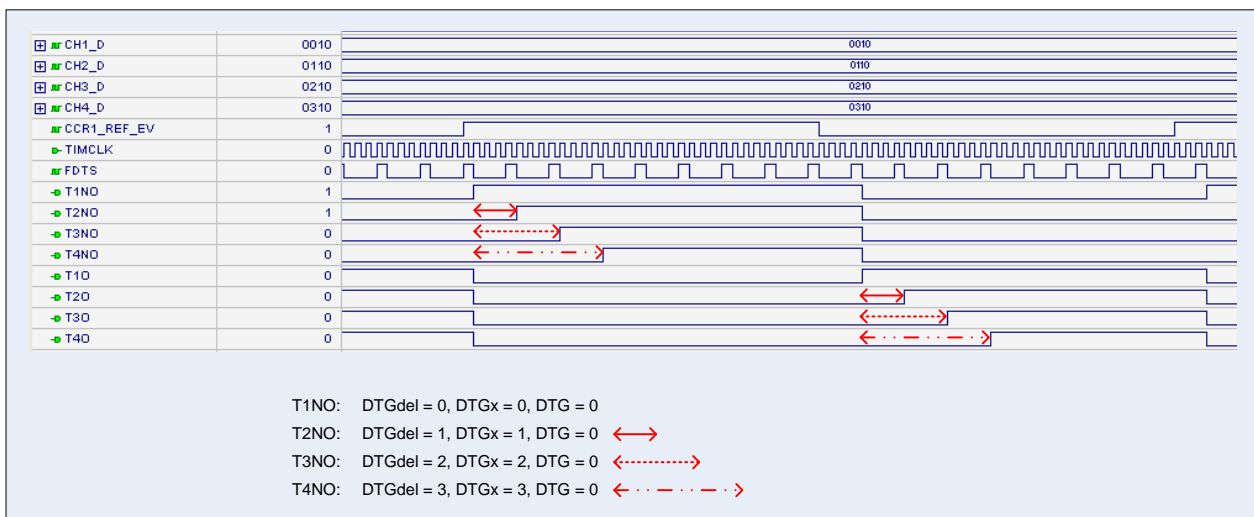
Рисунок 50 – Диаграмма работы схемы DTG
