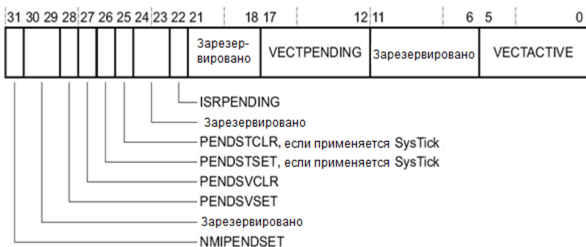
Рисунок 123 – Назначение разрядов регистра ICSR
