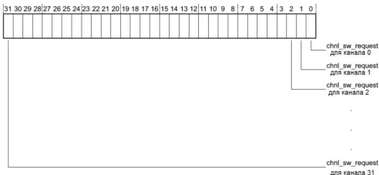
Рисунок 104 – Наименование разрядов регистра chnl_sw_request
