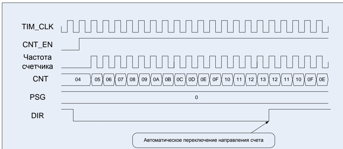
Рисунок 30 – Диаграммы работы таймера, счет вверх/вниз, сначала вверх
