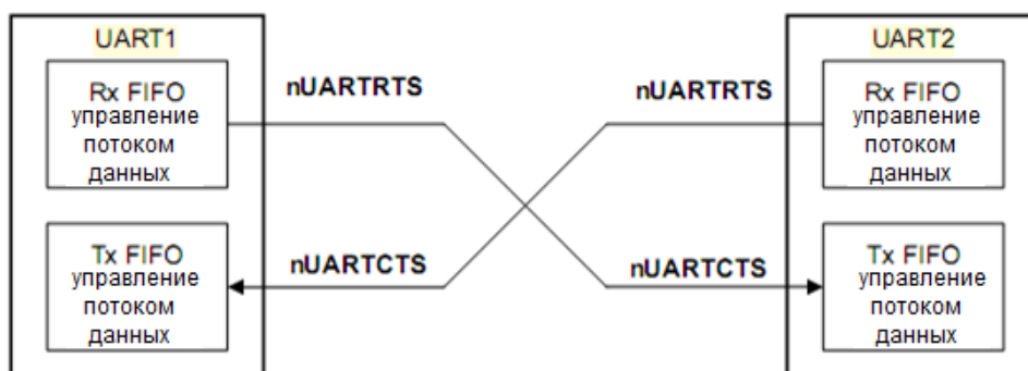
Рисунок 82 – Взаимодействие двух устройств последовательной связи с аппаратным управлением потоком данных
