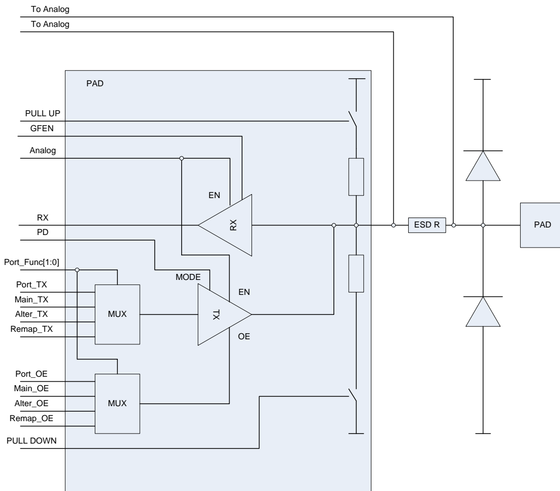
Рисунок 26 – Порты ввода/вывода
