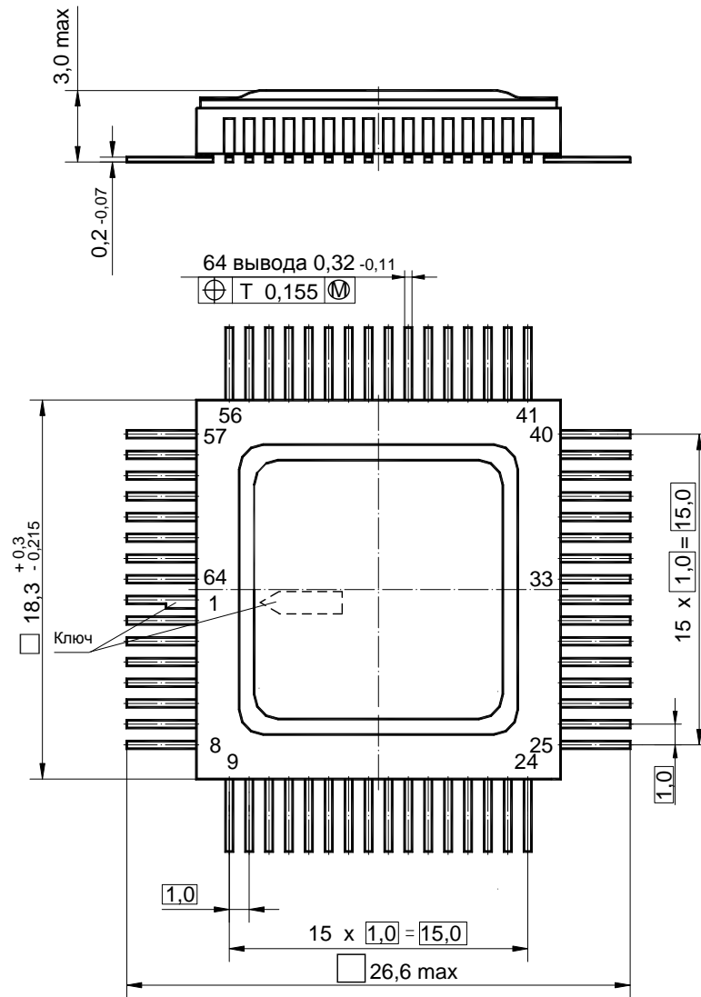
Рисунок 129 – Корпус N18.64-1B
