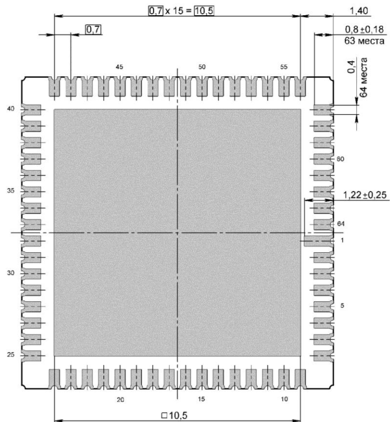
Рисунок 130 – Корпус 5153.64-1
