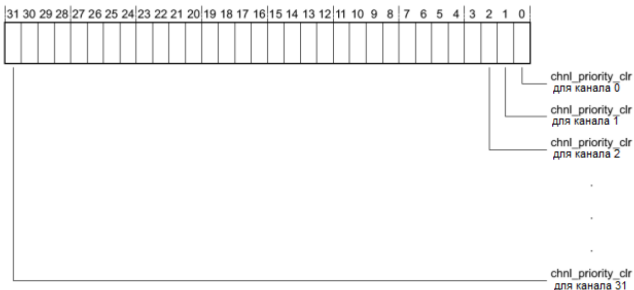
Рисунок 114 – Наименование разрядов регистра chnl_priority_clr
