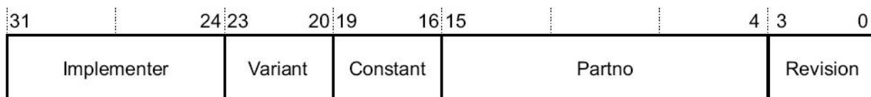
Рисунок 122 – Назначение разрядов регистра CPUID
