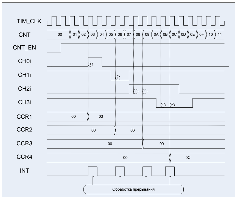
Рисунок 53 – Диаграммы примера работы в режиме захвата
