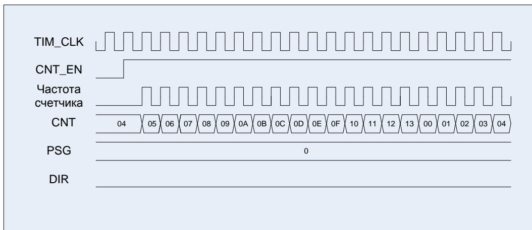
Рисунок 28 – Диаграммы работы таймера, счет вверх от 0 до 0x0013, стартовое значение 0x0004
