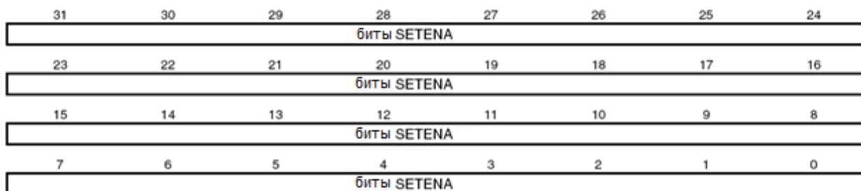
Рисунок 117 – Распределение битов регистра ISER
