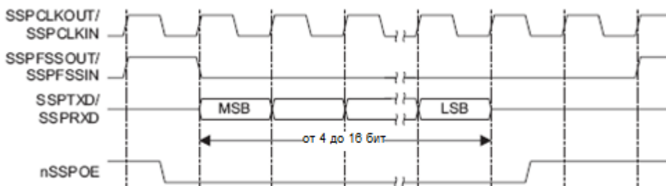
Рисунок 62 – Формат синхронного обмена протокола SSI фирмы Texas Instruments (единичный обмен)
