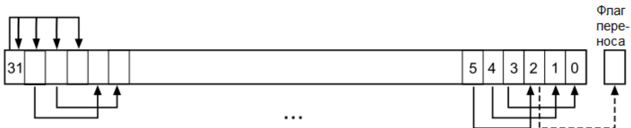
Рисунок 16 – Инструкция ASR #3
