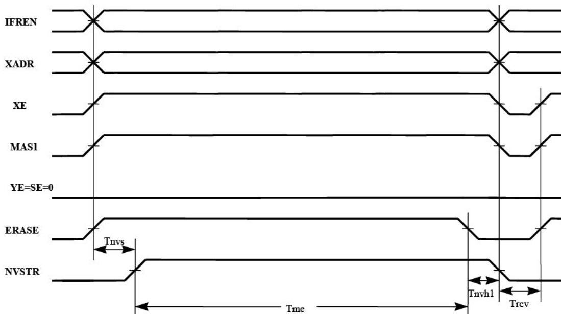
Рисунок 10 – Временная диаграмма стирания памяти
