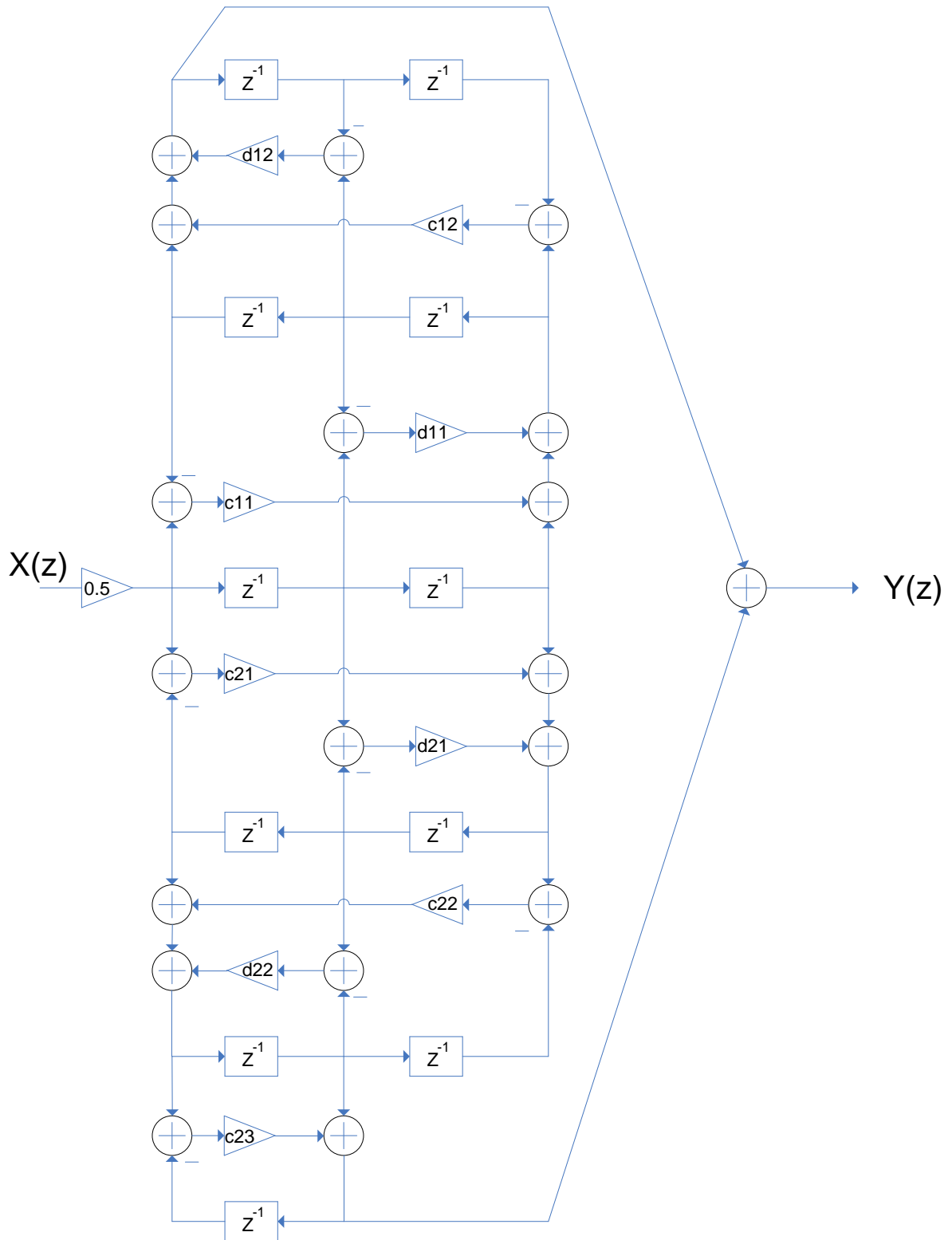
Рисунок 21 – Структурная схема IIR фильтра
