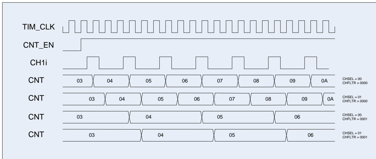
Рисунок 40 – Диаграмма внешнего тактирования с разными вариантами фильтра
