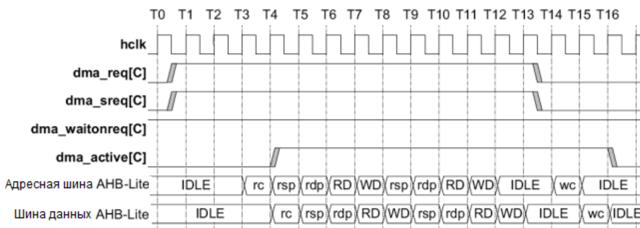
Рисунок 90 – Диаграмма работы контроллера ПДП при использовании периферией dma_waitonreq
