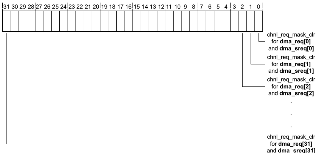
Рисунок 108 – Наименование разрядов регистра chnl_req_mask_clr
