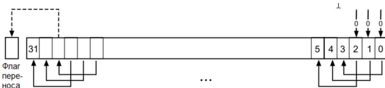
Рисунок 18 – Инструкция LSL \# 3
