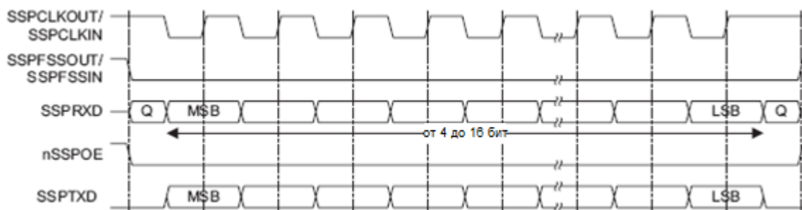
Рисунок 69 – Формат синхронного обмена протокола SPI фирмы Motorola, SPO=1, SPH=1
