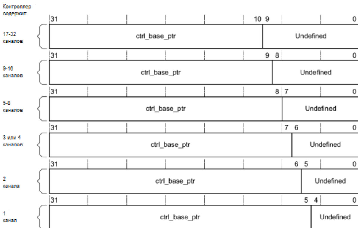
Рисунок 101 – Наименование разрядов регистра ctrl_base_ptr
