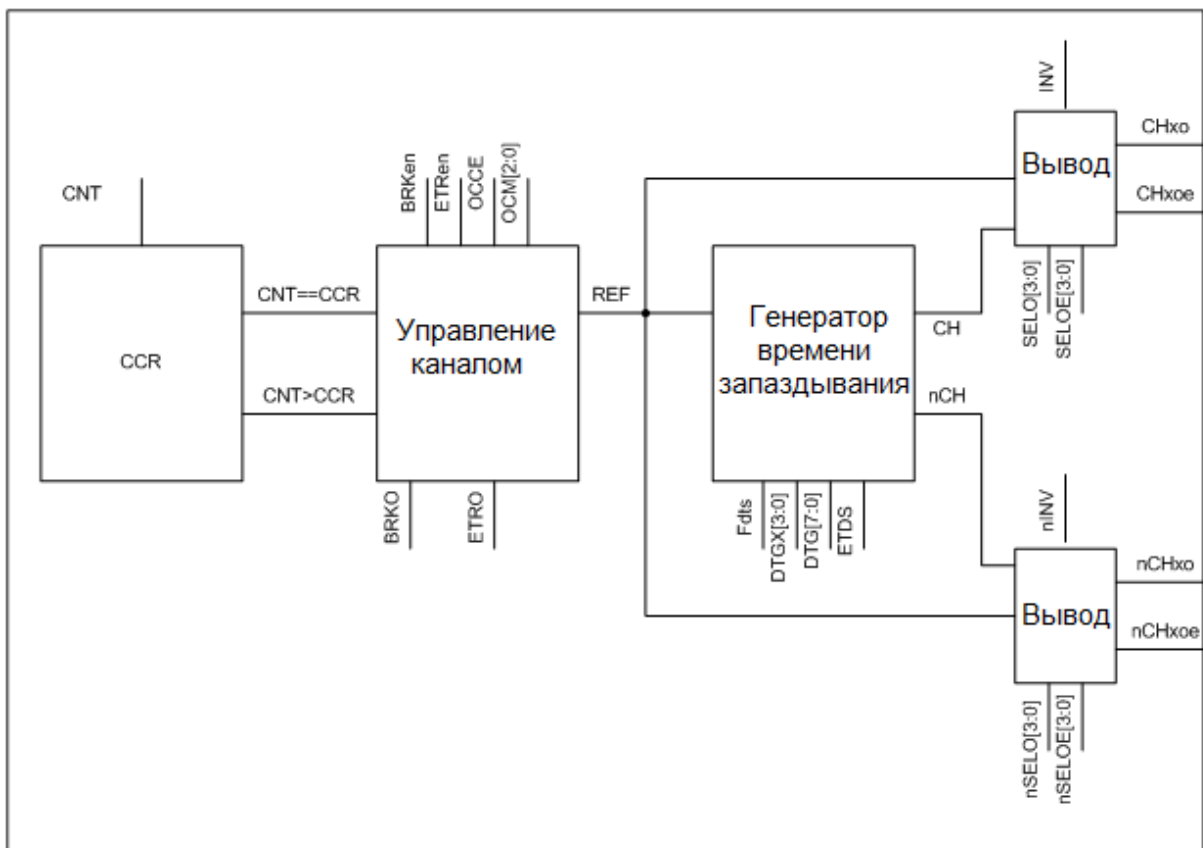
Рисунок 46 – Структурная схема блока сравнения
