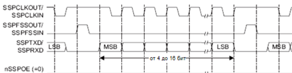
Рисунок 68 – Формат синхронного обмена протокола SPI фирмы Motorola, SPO=1, SPH=0 (непрерывный обмен)
