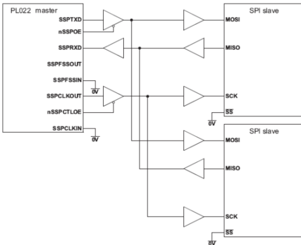
Рисунок 74 – Ведущее устройство PrimeCell SSP подключено к двум ведомым, поддерживающим протокол SPI
