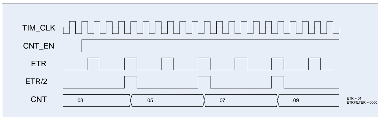
Рисунок 43 – Диаграмма тактирования сигналом со входа ETR
