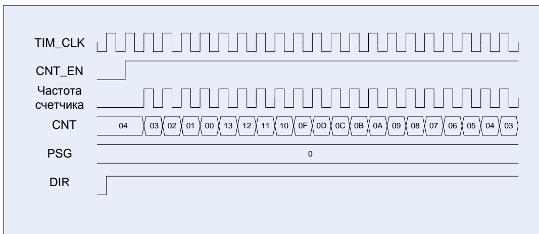
Рисунок 29 – Диаграммы работы таймера, счет вниз от 0x0013 до 0, стартовое значение 0x0004
