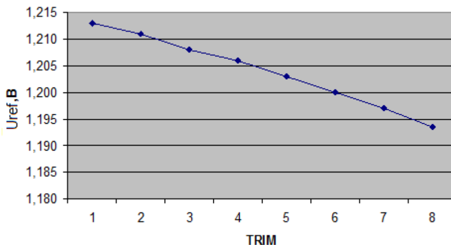
Рисунок 56 – Зависимость источника опорного напряжения от подстройки
