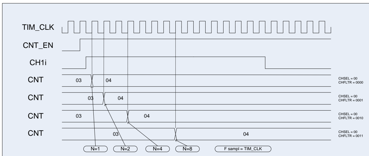
Рисунок 41 – Диаграмма внешнего тактирования с разными вариантами фильтра
