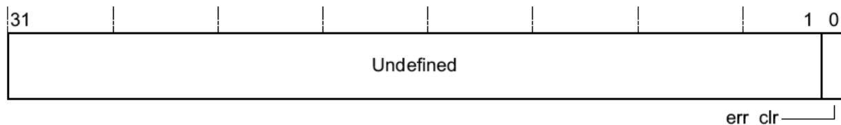
Рисунок 115 – Наименование разрядов регистра err_clr
