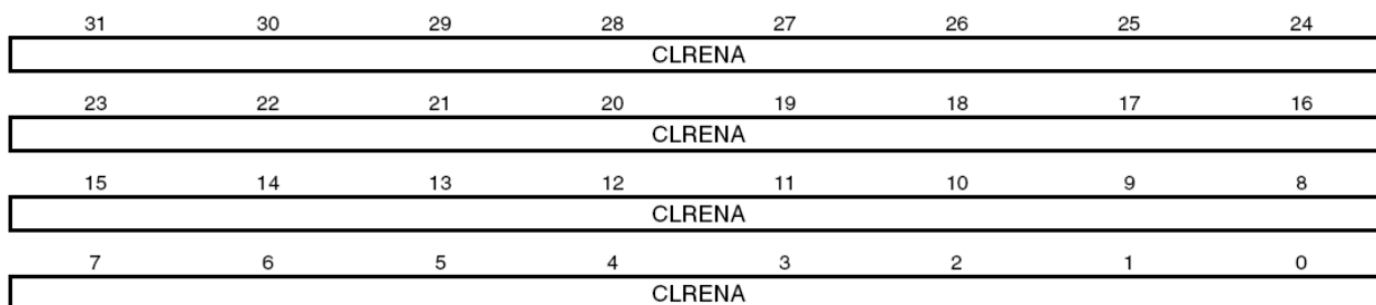
Рисунок 118 – Распределение битов регистра ICER
