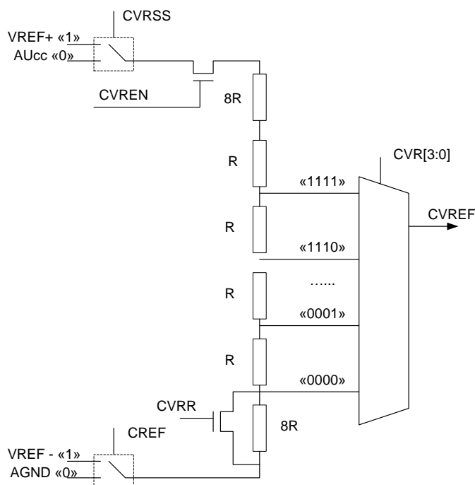
Рисунок 60 – Структура блока формирования CVREF
