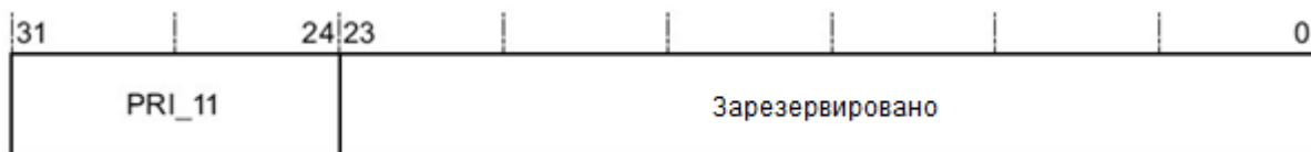
Рисунок 127 – Назначение разрядов регистра
