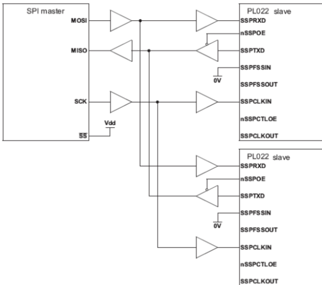
Рисунок 75 – Ведущее устройство, поддерживающее протокол SPI подключено к двум ведомым модулям PrimeCell SSP
