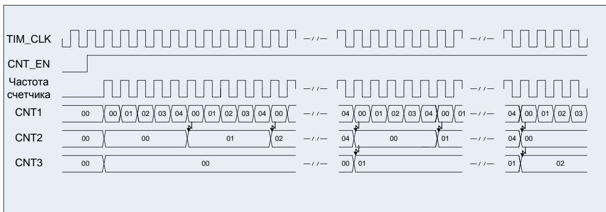
Рисунок 37 – Диаграммы работы трех таймеров в каскаде
