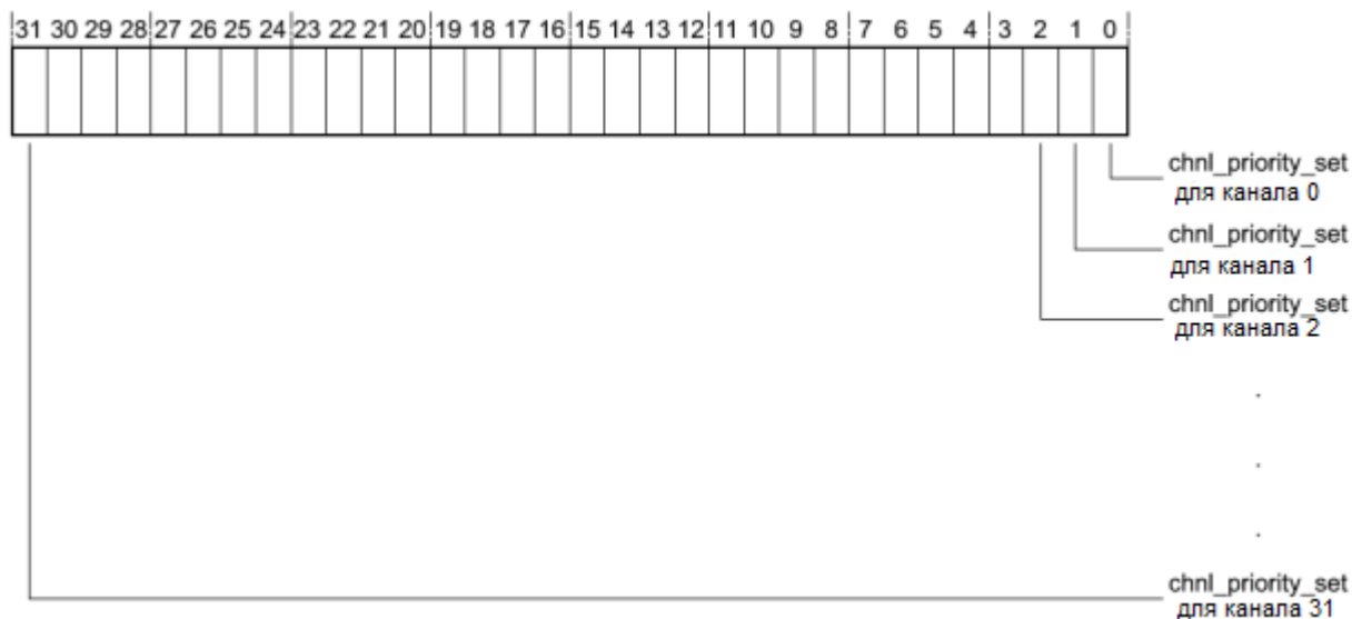
Рисунок 113 – Наименование разрядов регистра chnl_priority_set
