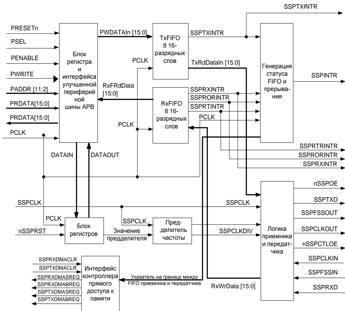
Рисунок 61 – Структурная схема модуля SSP
