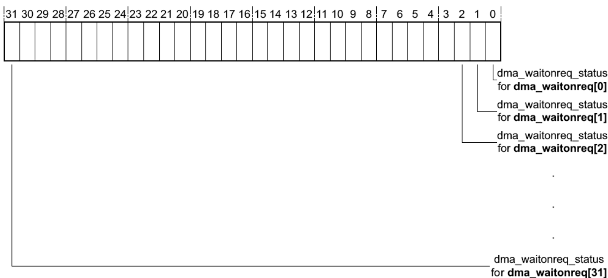
Рисунок 103 – Наименование разрядов регистра dma_waitonreq_status
