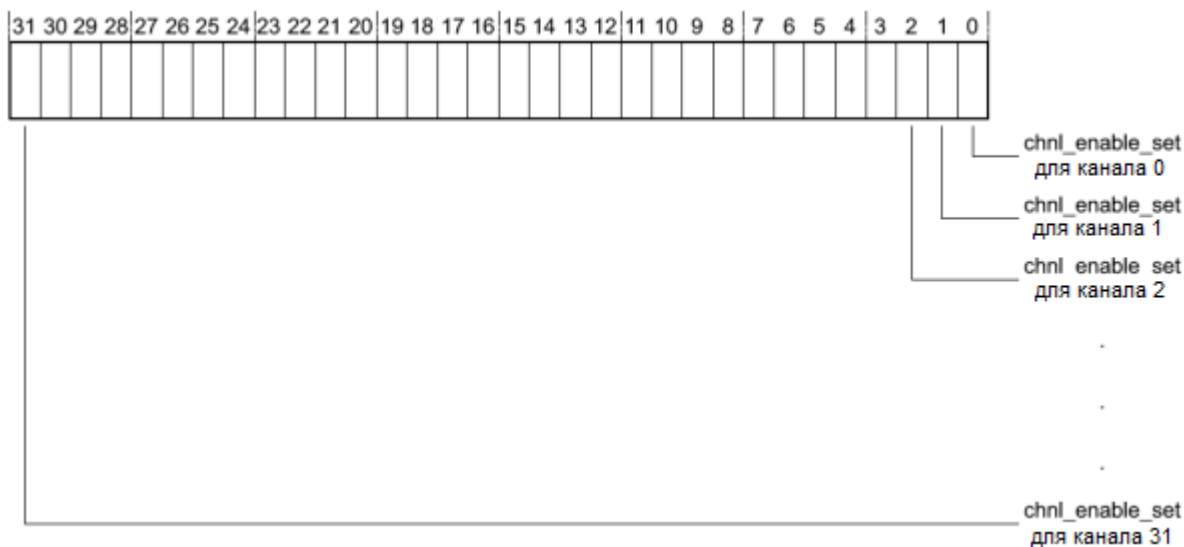
Рисунок 109 – Наименование разрядов регистра chnl_enable_set
