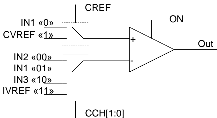
Рисунок 59 – Схема компаратора
