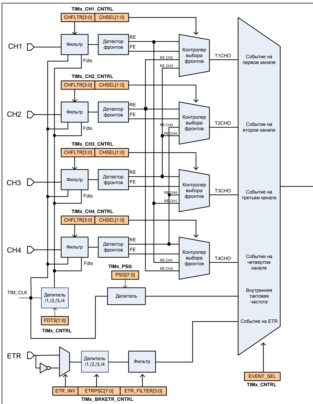
Рисунок 32 – Структурная схема формирования события для счета
