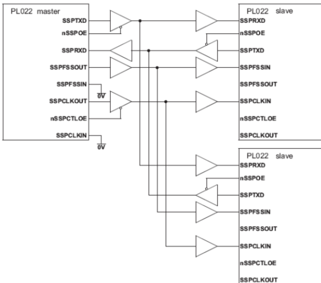
Рисунок 73 – Ведущее устройство PrimeCell SSP подключено к двум ведомым
