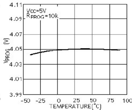
再充电电压门限与温度的关系曲线
