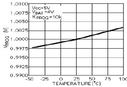
稳定输出（浮充）电压与温度的关系曲线
