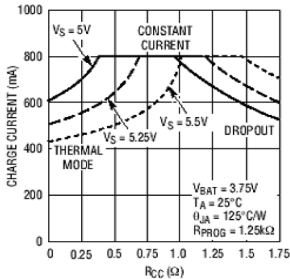
图 4：充电电流与 R_{CC} 的关系曲线
