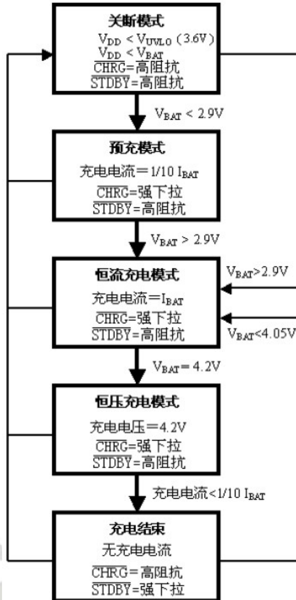
图1：一个典型充电循环的状态图
