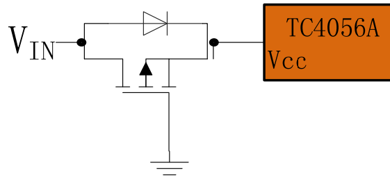
图 5:低损耗输入反向极性保护
