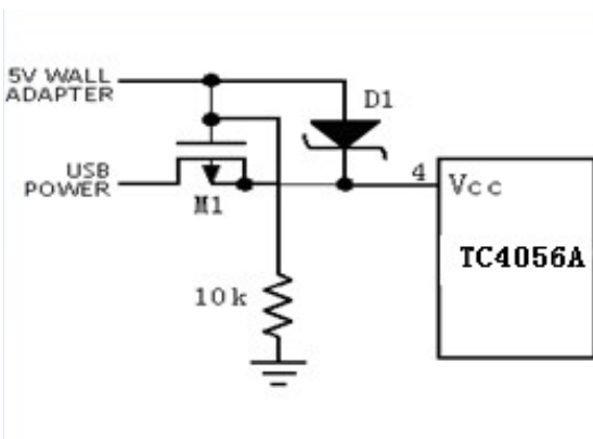
适合同时应用USB接口和墙上适配器充电
