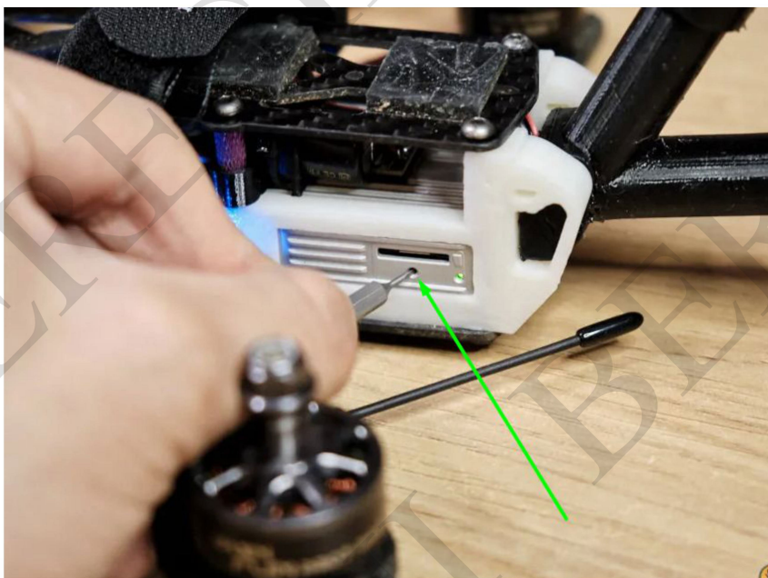
Кнопка біндингу на Air Unit (потріна шпилька)
